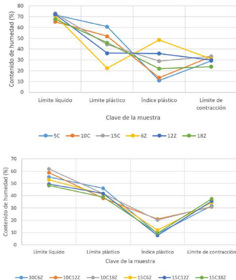
Figura 4.4 Variación de los límites de Atterberg a diferentes cantidades de cal y zeolita.
