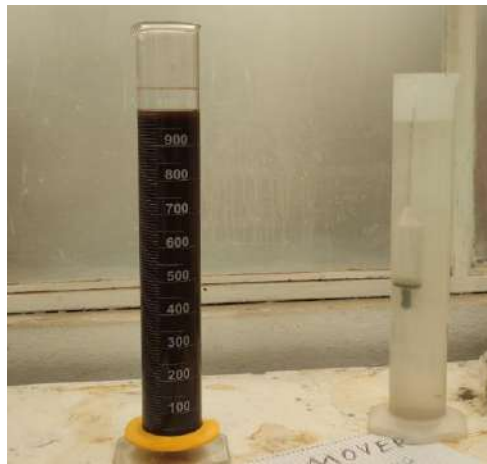
Figura 3.11 Probeta con solución de suelo e hidrómetro para medición.
