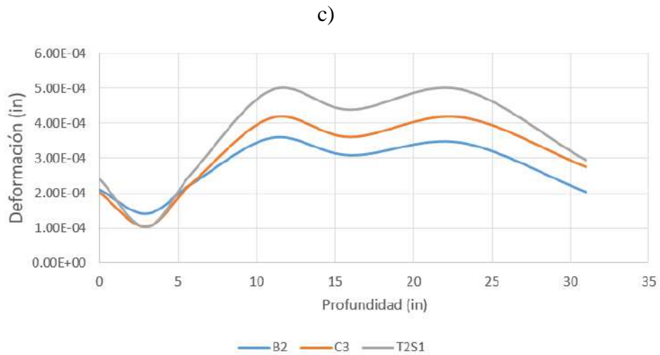
Figura 4.7 Variación de esfuerzos y deformaciones en un pavimento con subbase de banco Fuente: Elaboración propia.
