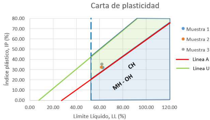
Figura 4.3 Carta de plasticidad de Casagrande y coordenadas del suelo muestreado.
