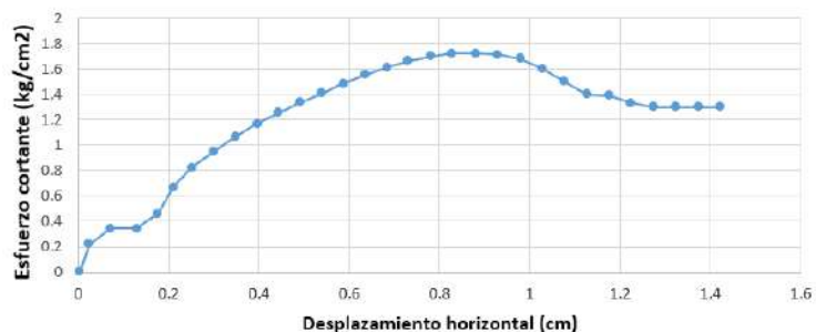
Esfuerzo cortante - Desplazamiento horizontal (E2)
