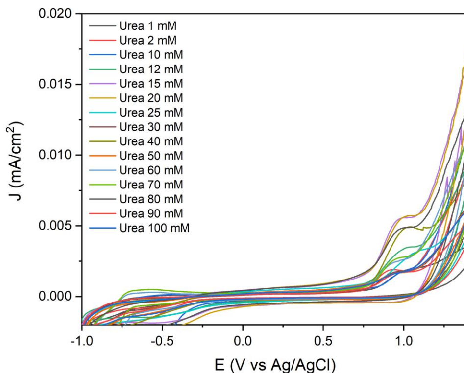
Figura 7.23. Voltametrías cíclicas de electrodo de carbón vítreo modificado con tinta catalítica de Vulcan/IrNP's para soluciones de urea a diferentes concentraciones, de 1 mM a 100 mM.
