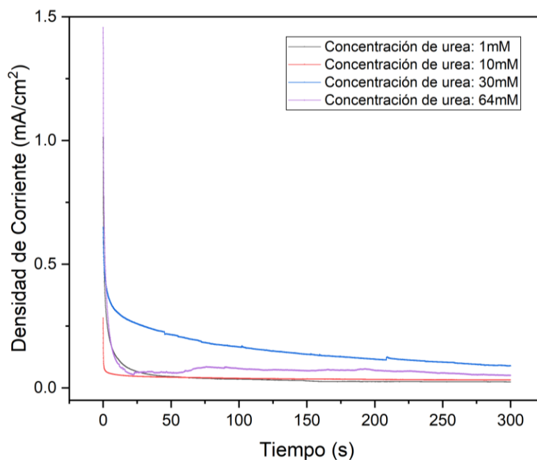
Figura 7.31. Cronoamperometría a 1 V en celda de combustible microfluídica para un electrodo Vulcan/IrNP's/ureasa en solución de urea: 1 mM, 10 mM, 30 mM y 64 mM.
