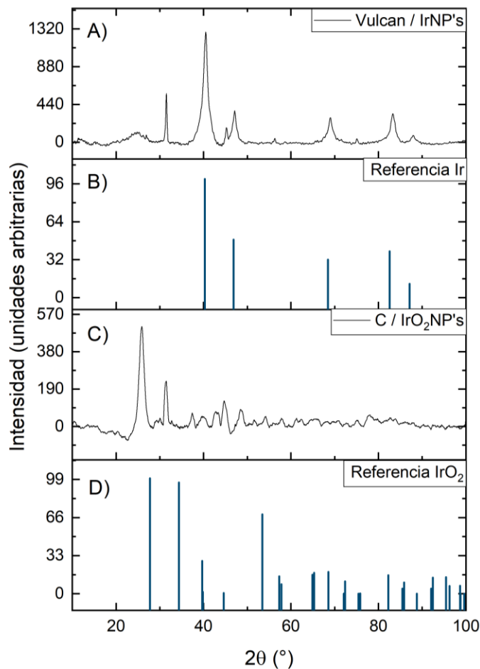
Figura 7.5. Difractogramas de rayos X obtenidos de los sistemas sintetizados, comparados con los difractogramas de Iridio (B) y Dióxido de Iridio (D) obtenidos de Materials Project.
