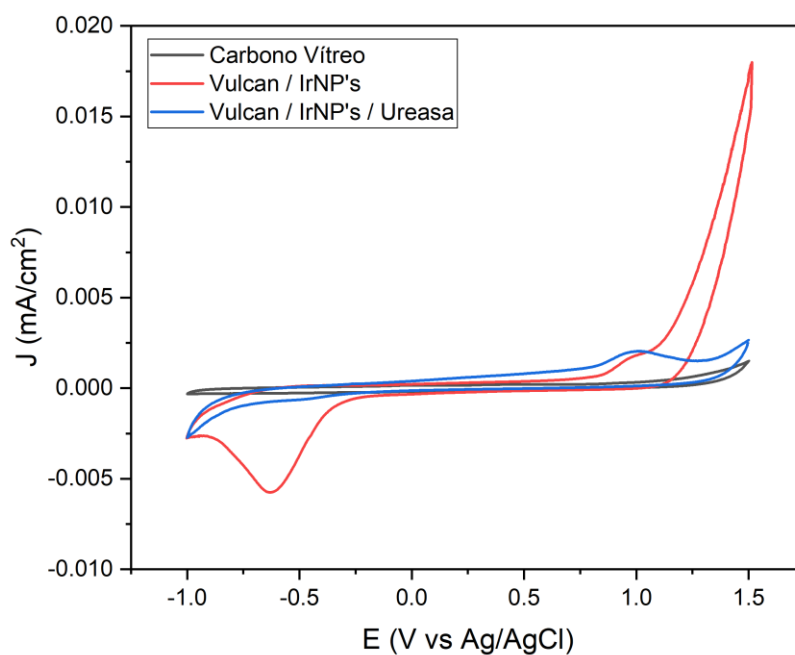
Figura 7.16. Voltametría cíclica (CV) del electrodo propuesto de carbón vulcan decorado con IrNP's y ureasa inmovilizada en una solución de urea 10 mM graduada con tampón pH 7.0 contra una curva de control de carbono vítreo y el material sin inmovilización enzimática.
