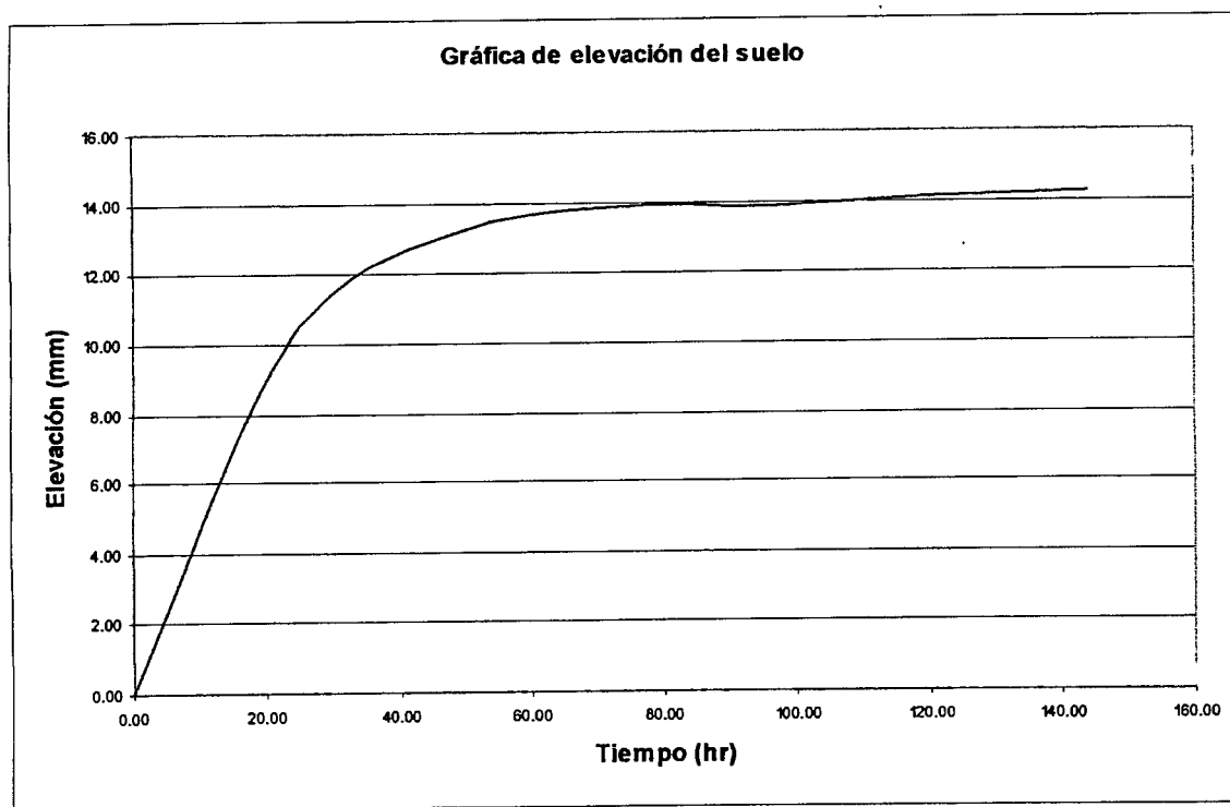
Fig. 4.5 Gráfica de expansión del material con respecto al tiempo.
