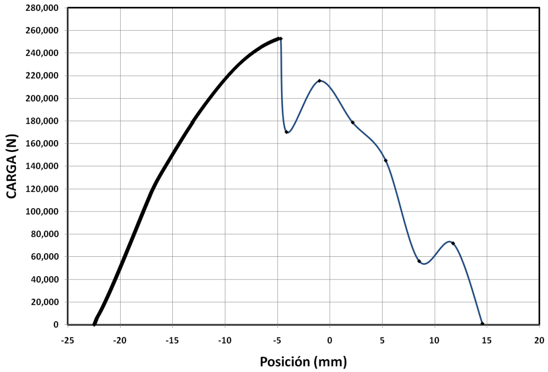
Figura 4.3 Gráfico de Posición/Carga para la probeta EN-20110401-008
