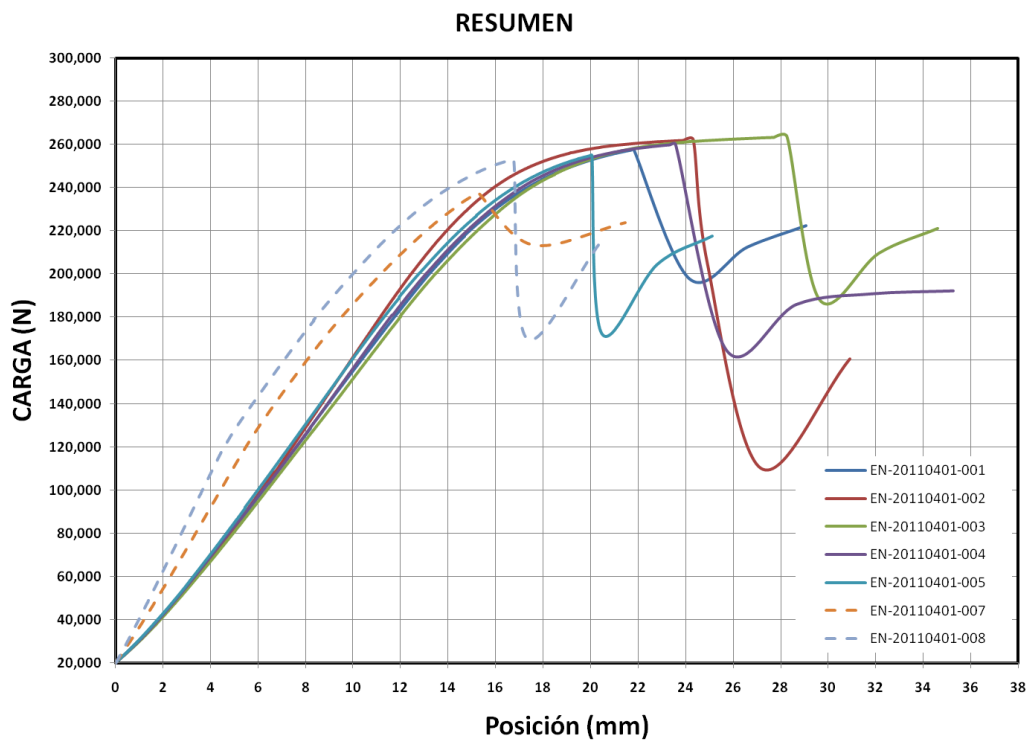
Figura 4.5 Resumen de las pruebas de Tensión y Fatiga-Tensión.
