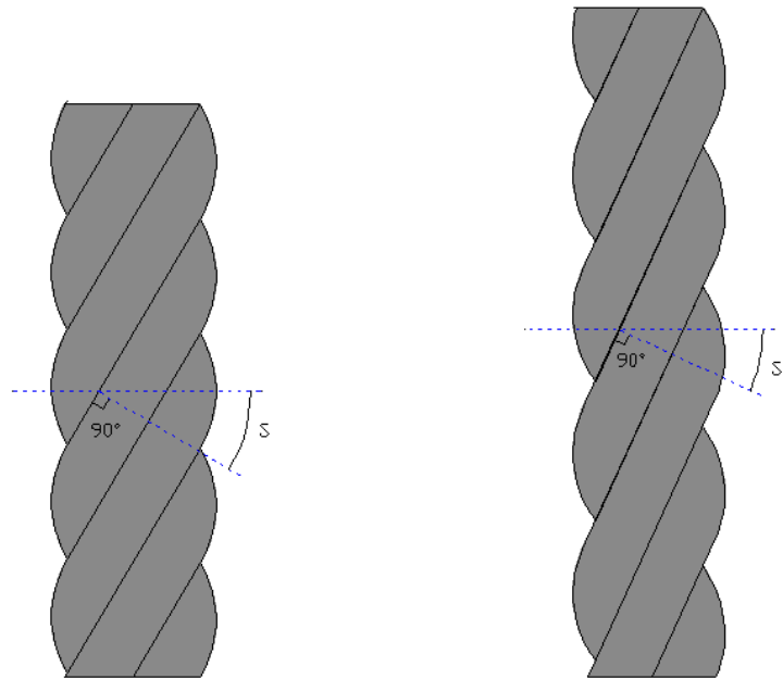
Figura 4.15 Variación del ángulo de ruptura
