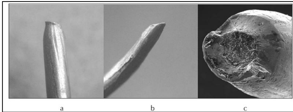
Figura 2.18 Fallas en alambres de torones por sobrecarga
