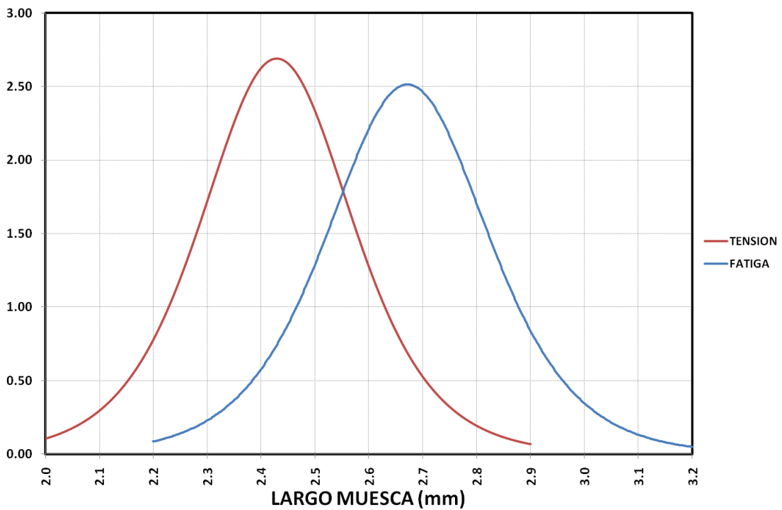
Figura 4.18 Comparativa del daño causado por la incrustación de la mordaza a lo largo
