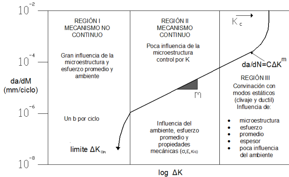
Figura 2.32 Curva de propagación de grieta por fatiga.
