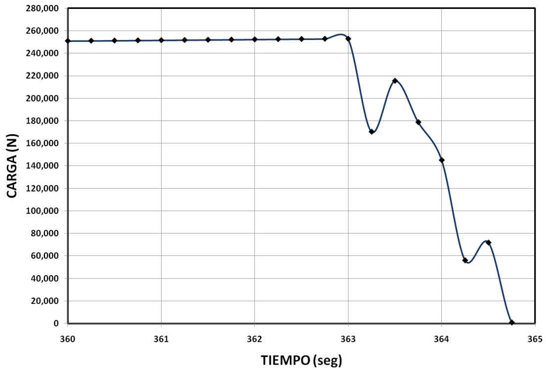
Figura 4.4 Gráfico de Tiempo/Carga para la probeta EN-20110401-008
