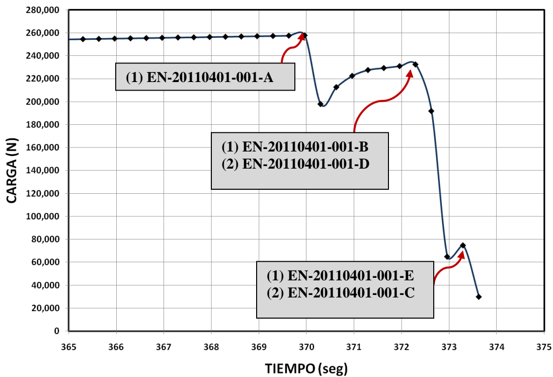
Figura 4.26 Curva de Tiempo/Carga con secuencia de ruptura de la probeta EN-20110401-001
