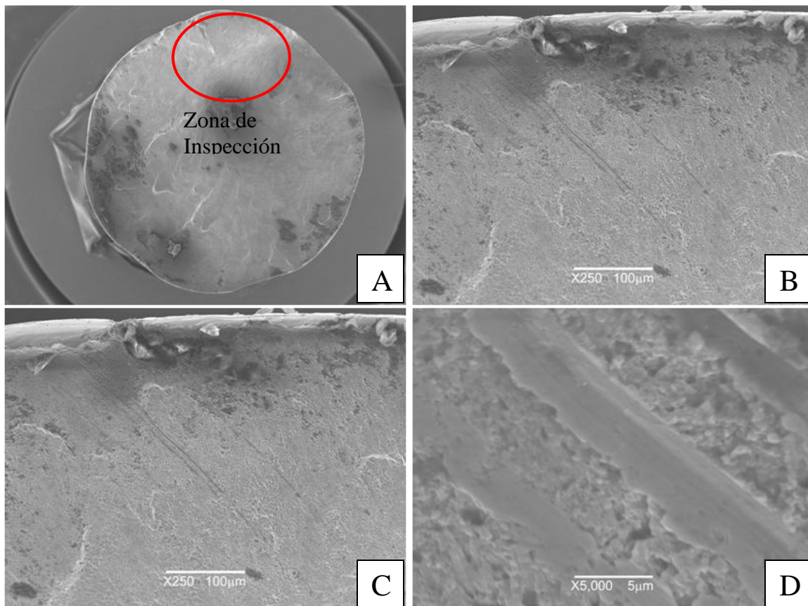
Figura 4.19 Fractografías del alambre EN-20110401-007-E1
