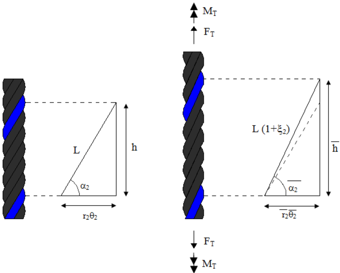
Figura 2.24 Torón sujeto a fuerza axial
