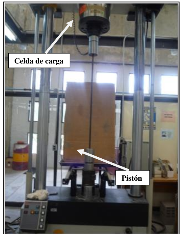
Figura 3.7 Montaje del dispositivo en la máquina servo hidráulica Instron
