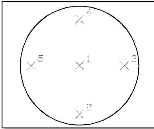
Figura 3.13 Secuencia y posición de las indentaciones
