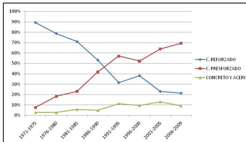
Figura 2.1 Tendencias en la construcción de puentes en México por tipo de superestructura Fuente: Base de Datos del Sistema de Puentes Mexicano SIPUMEX 2010.
