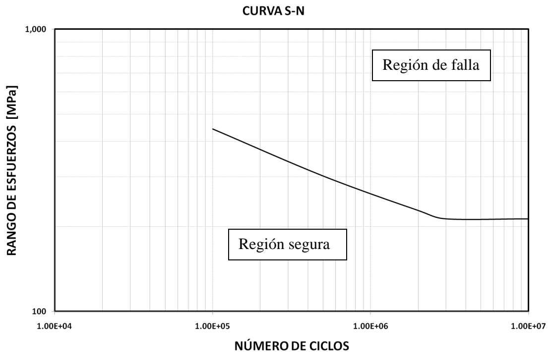
Figura 3.2 Recomendaciones del PTI para las pruebas de calidad a la fatiga.
