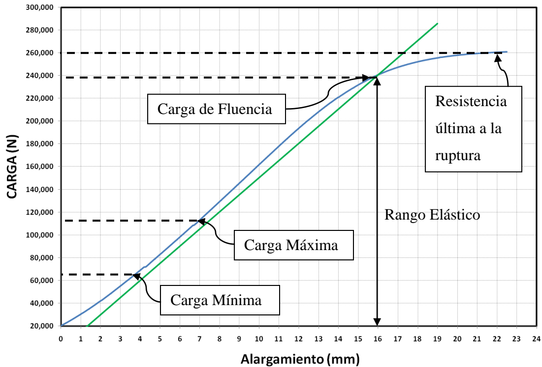
Figura 3.5 Comportamiento típico de un torón en la prueba de carga.
