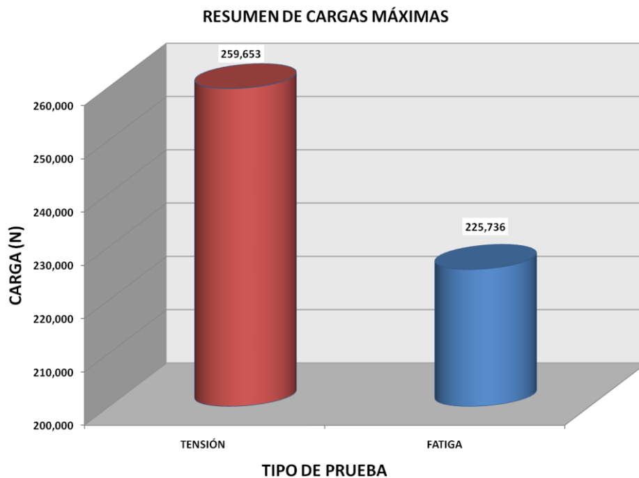
Figura 4.6 Comparativa de Cargas últimas resistentes por tipo de prueba
