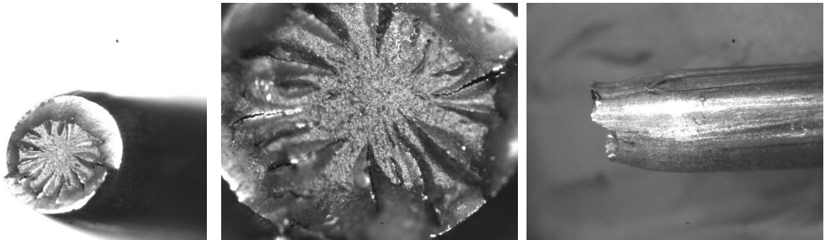
Figura 4.10 Fractografías del alambre EN-20110401-001-D
