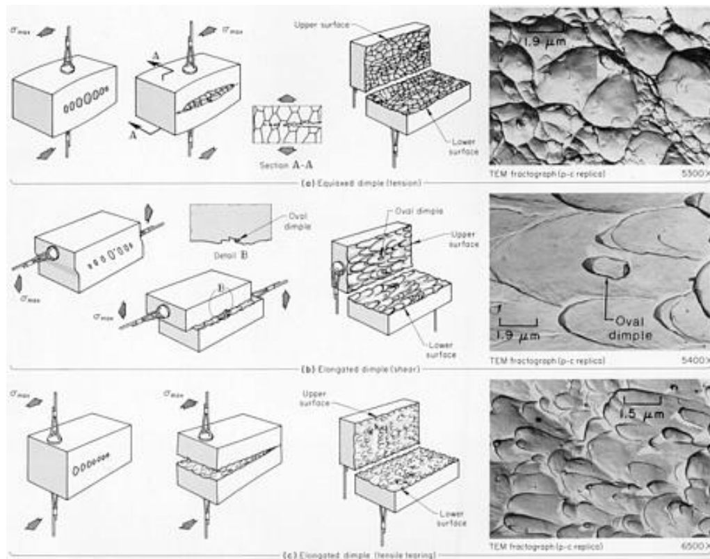
Figura 2.30 Formación de cavidades de acuerdo al modo de carga
