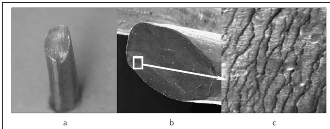
Figura 2.20 Fractura a 45° por fatiga en un alambre, a) Vista frontal, b) detalle del patrón de fractura y c) acercamiento de las estrías por fatiga.
