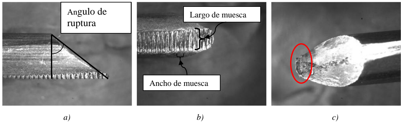
Figura 4.13 Imágenes de la fractura diagonal en un alambre
