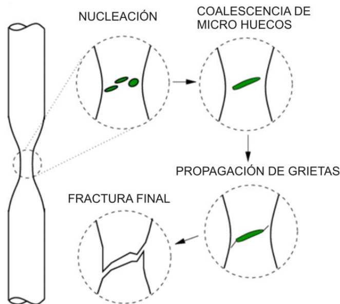
Figura 2.28 Proceso de ruptura dúctil
