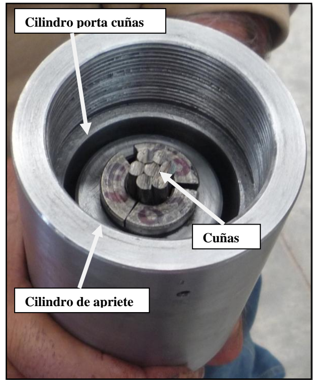
Figura 3.6 Montaje del torón en el sistema de anclaje.
