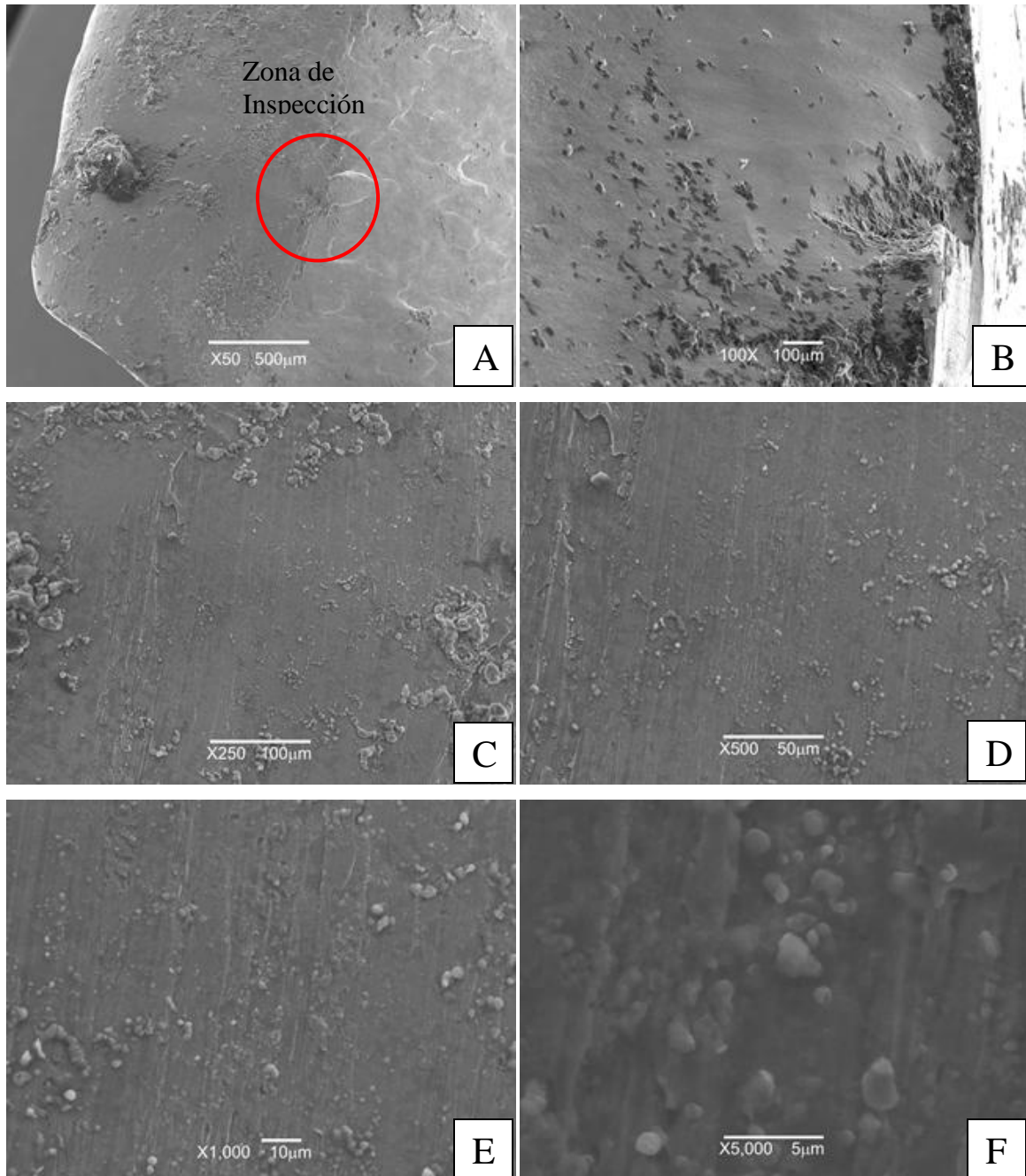
Figura 4.23 Fractografías del alambre EN-20110401-008-D2
