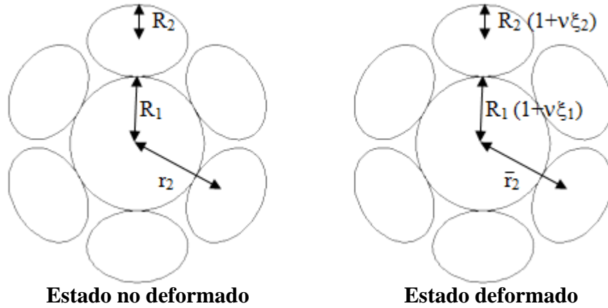
Figura 2.23 Sección transversal de un torón de capa simple
