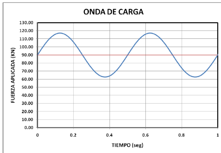
Figura 10.- Onda de carga de la prueba de fatiga.
