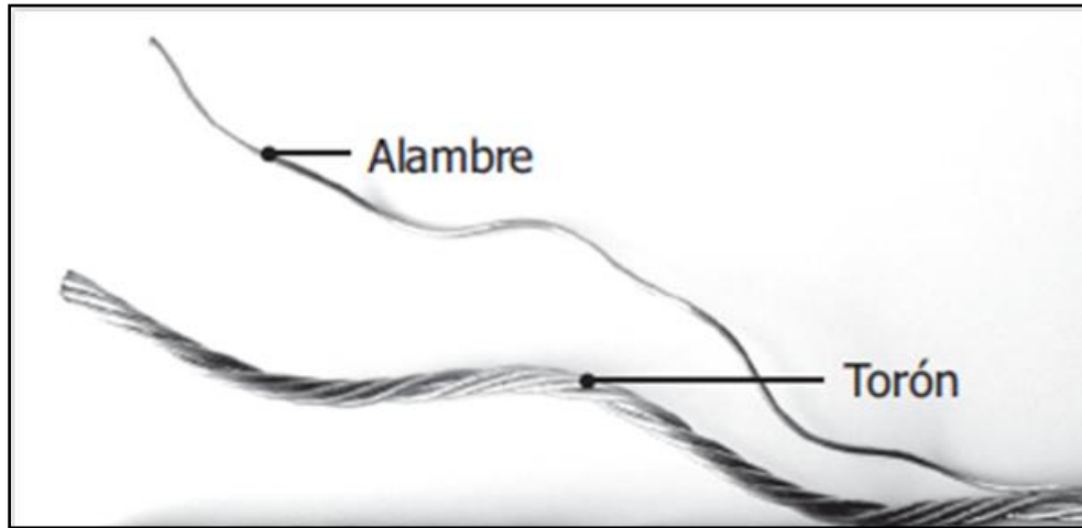
Figura 2.16 Constitución de los torones de acero Fuente: Manual de Emcables.
