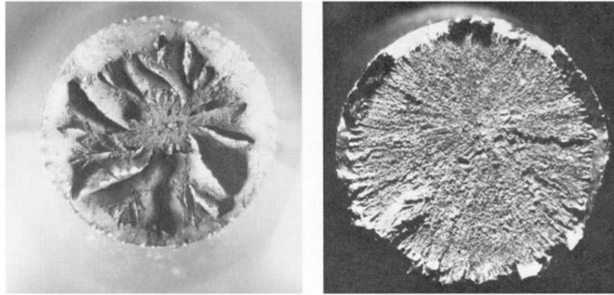
Figura 2.33 Elemento fracturado por sobrecarga de tensión
