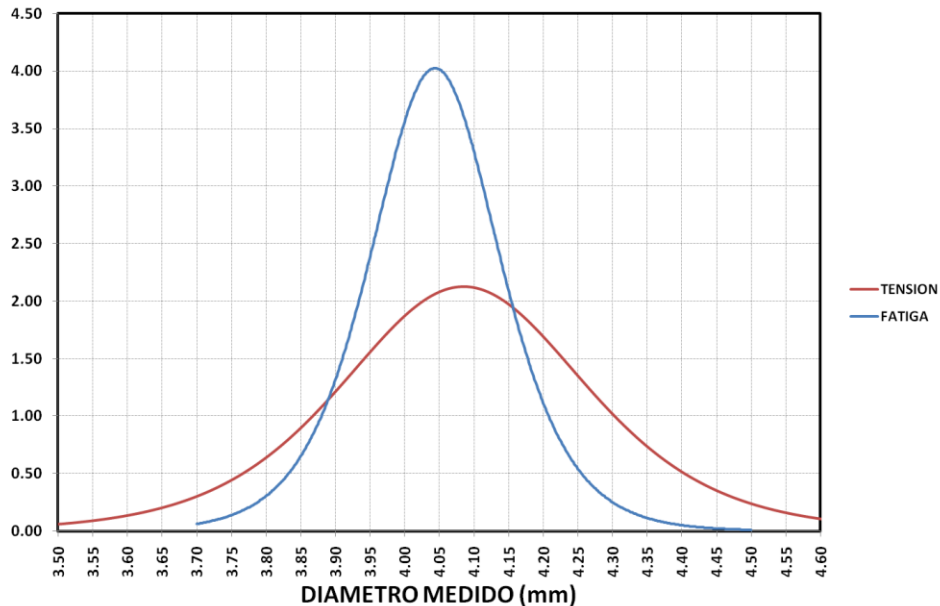
Figura 4.12 Comparativa del diámetro reducido por estricción
