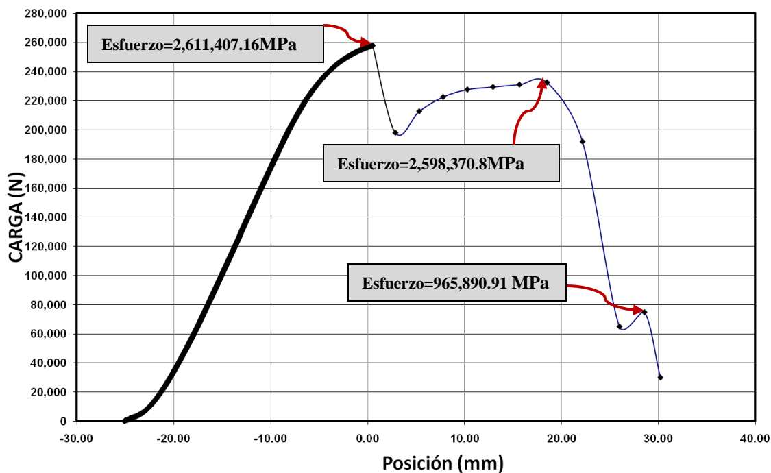
Figura 4.25 Curva de Posición/Carga con esfuerzos de la probeta EN-20110401-001
