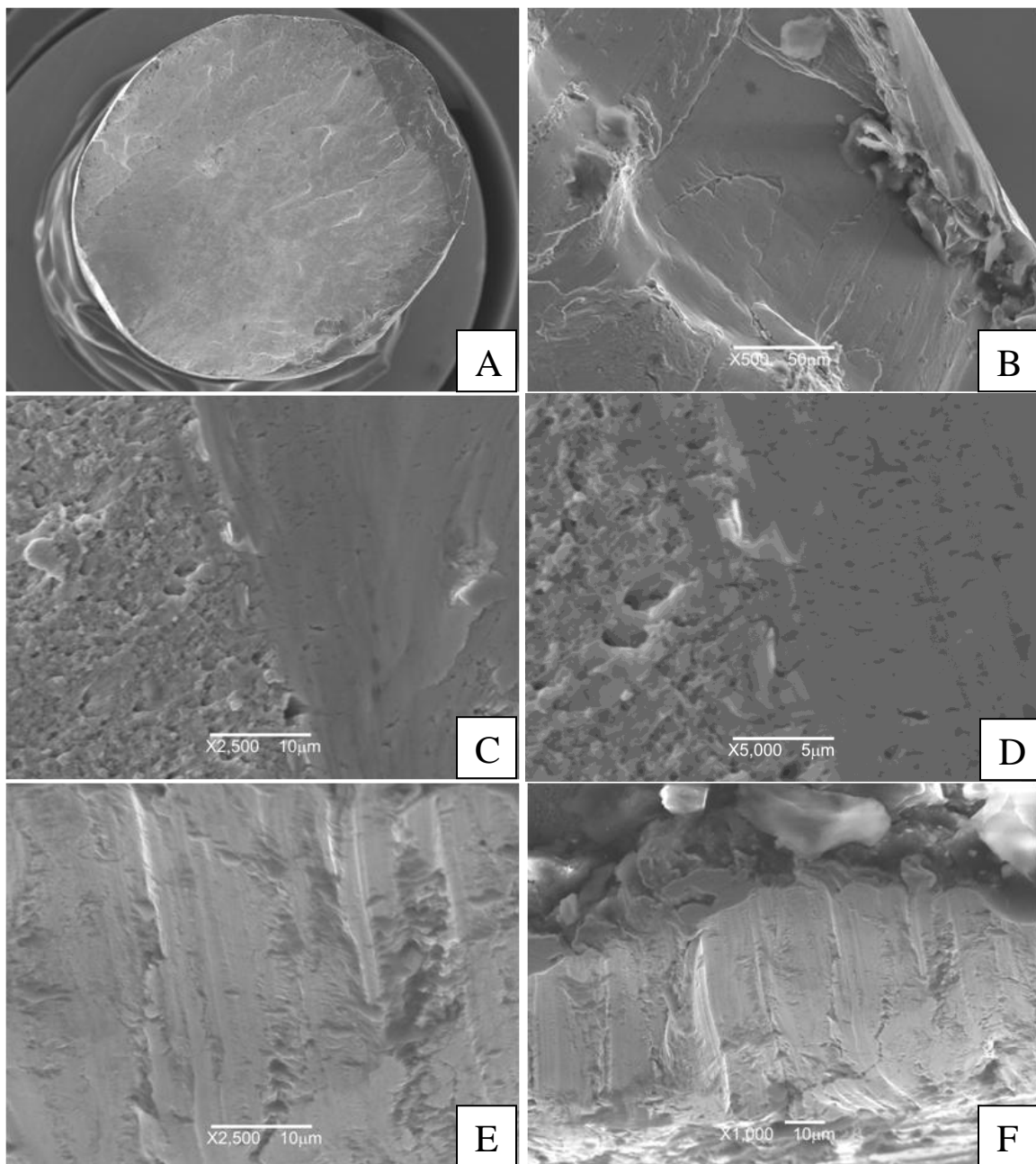
Figura 4.20 Fractografías del alambre EN-20110401-007-E2
