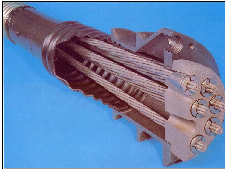
Figura 2.15 Dispositivo de anclaje Fuente: Stacy Johnson, 2006
