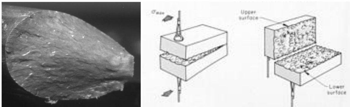
Figura 4.14 Ruptura de un elemento a tensión ante carga excéntrica
