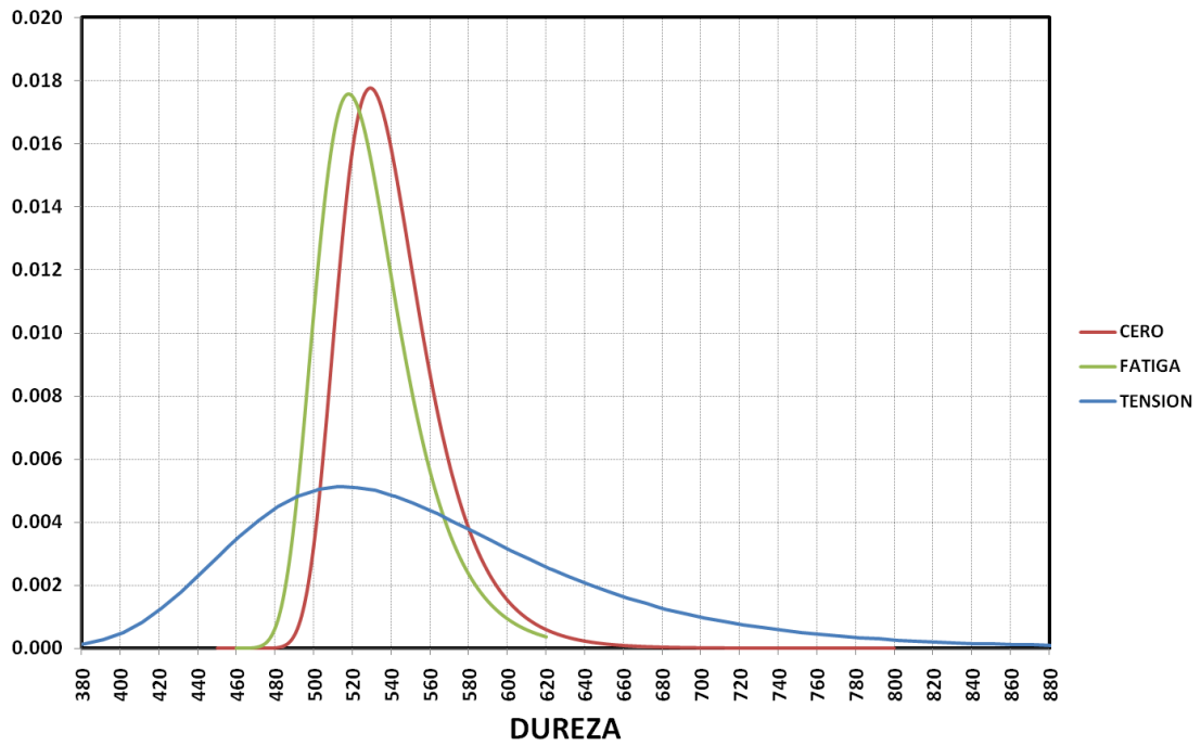
Figura 4.7 Comparativa de distribuciones de dureza por tipo de prueba
