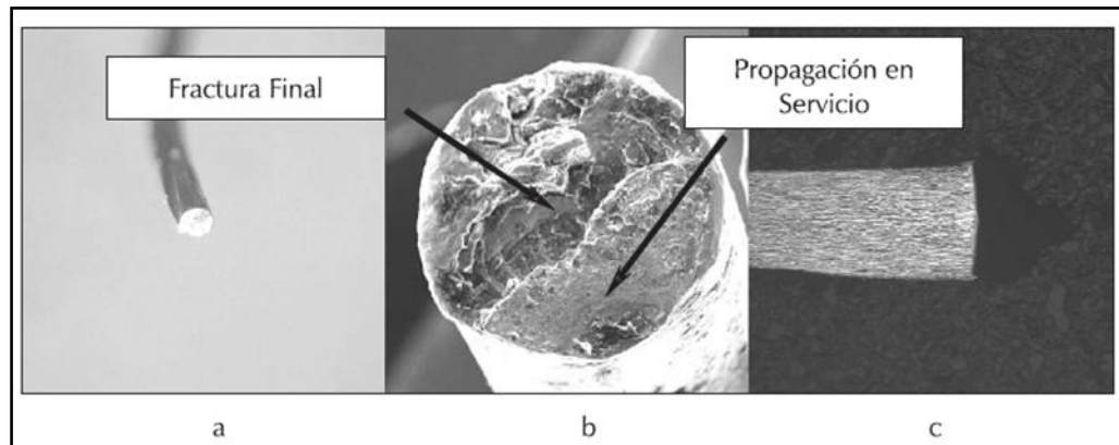
Figura 2.19 Fractura perpendicular al eje por fatiga en un alambre a) Vista frontal, b) vista con el microscopio electrónico de barrido (SEM) y c) Patrón de deformación por el proceso de manufactura.
