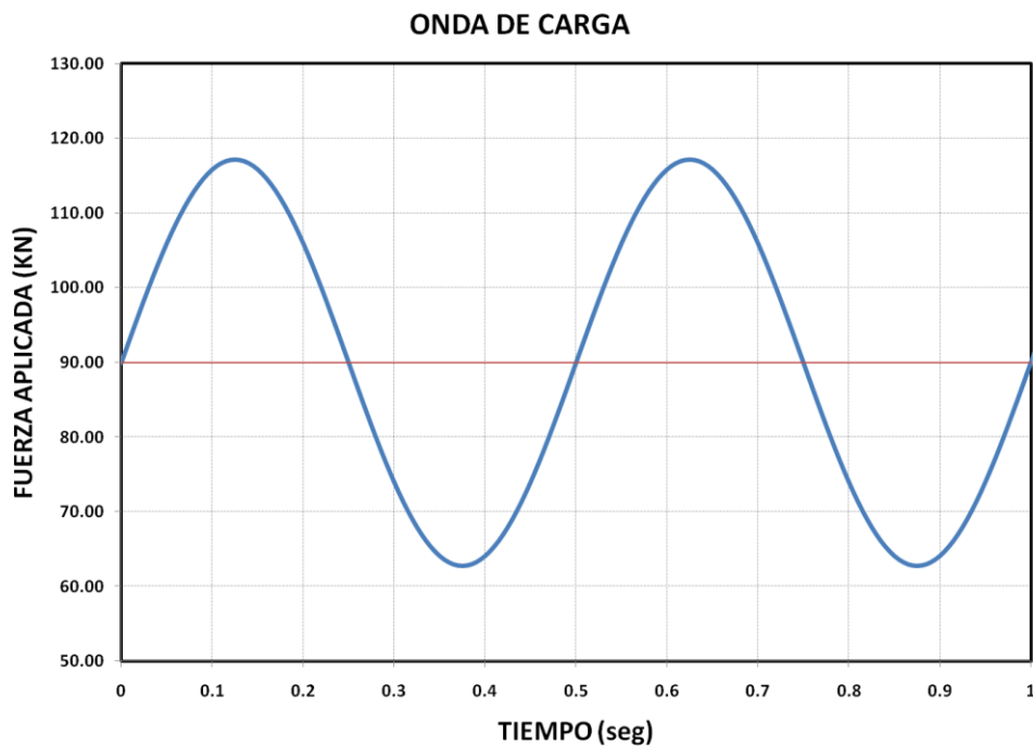
Figura 3.10 Onda de carga de la prueba de fatiga.
