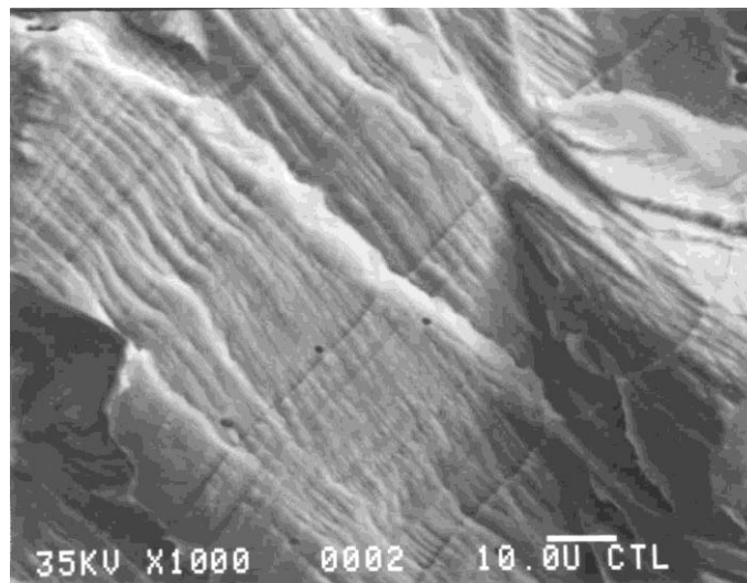
Figura 2.35 Marcas de estrías por fatiga ( http://www.corrosionlab.com/papers/techincal-brief-fatigue-failure.htm )
