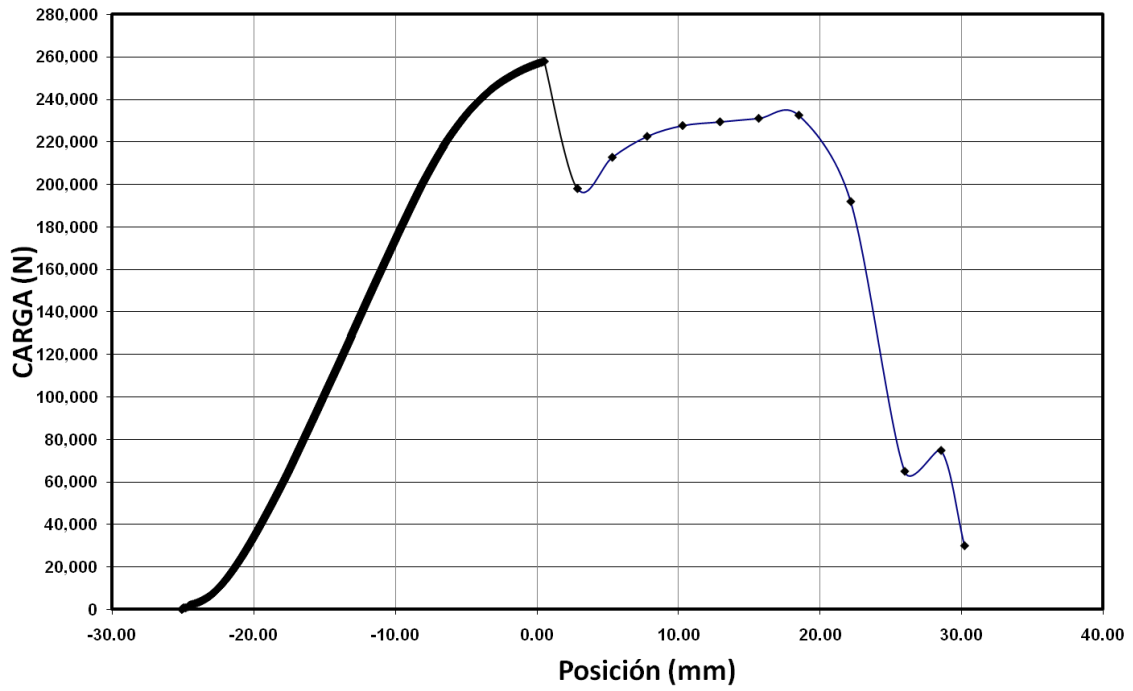
Figura 4.1 Gráfico de Posición/Carga para la probeta EN-20110401-001
