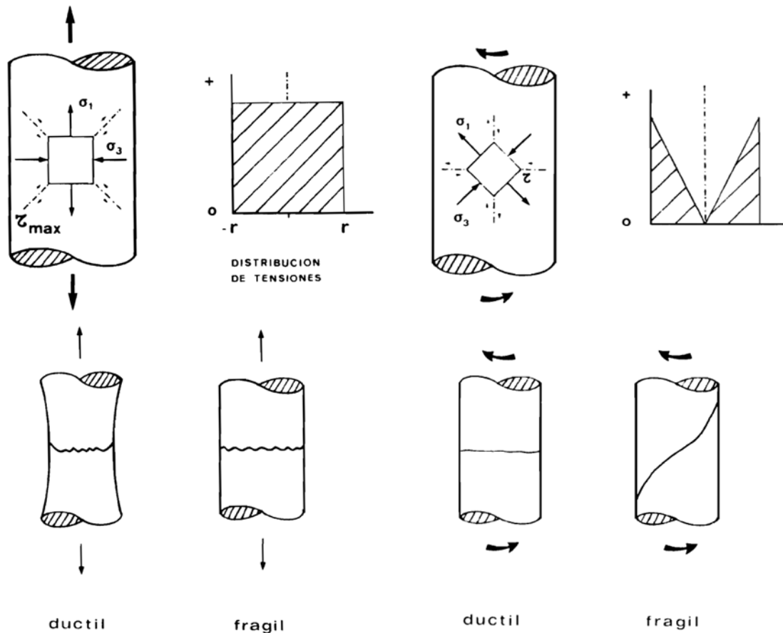
Figura 2.27 Fractura dúctil y frágil por tensión y por torsión.
