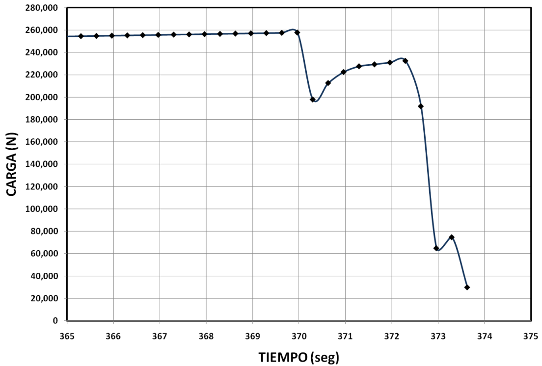
Figura 4.2 Gráfico de Tiempo/Carga para la probeta EN-20110401-001
