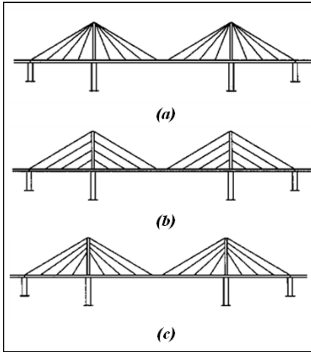
Figura 2.12 Tipo de arreglo de los tirantes: (a) Sistema de abanico, (b) Sistema de arpa(c) Sistema de semi-arpa Fuente: Samayoa,2005.
