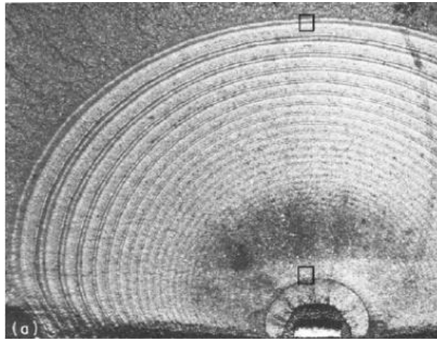
Figura 2.34 Marcas de playa en un elemento fracturado, ASM
