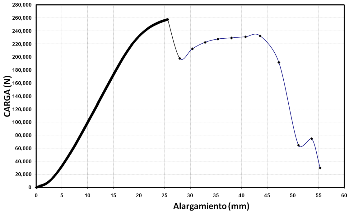
Figura 3.9 Curva típica de carga/posición.
