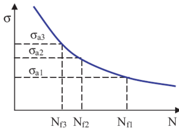
Figura 4.27 Curva de umbral de daño por fatiga
