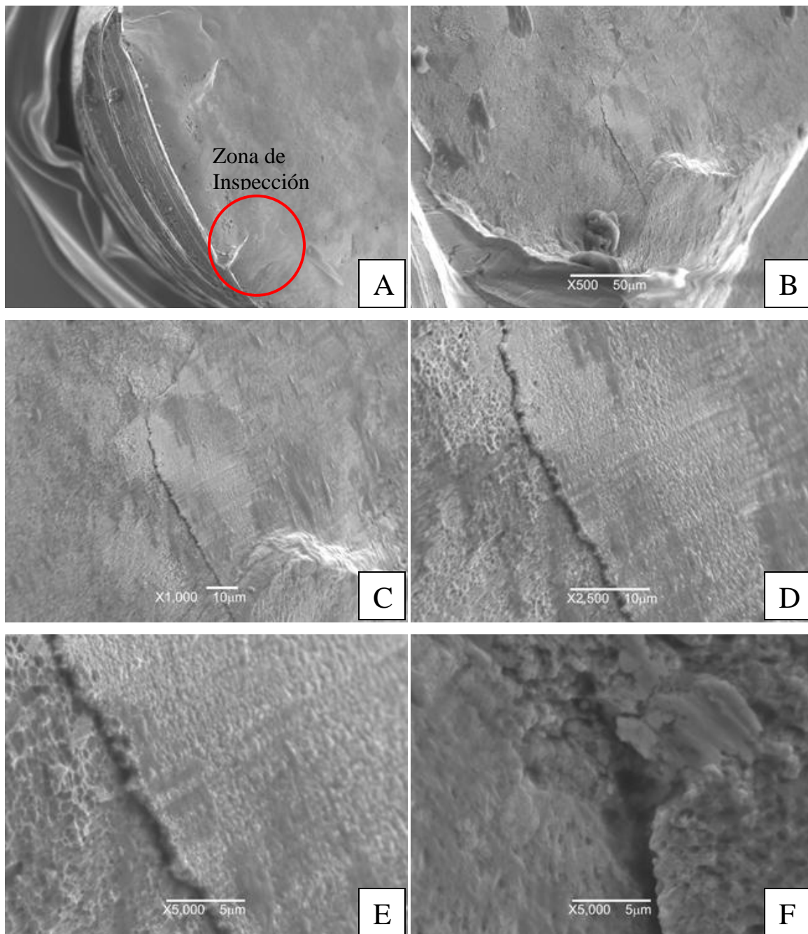
Figura 4.22 Fractografías del alambre EN-20110401-008-D1
