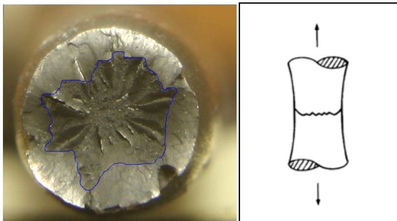
Figura 4.11 Medición de la zona fibrosa en un alambre con ruptura de Copa-Cono
