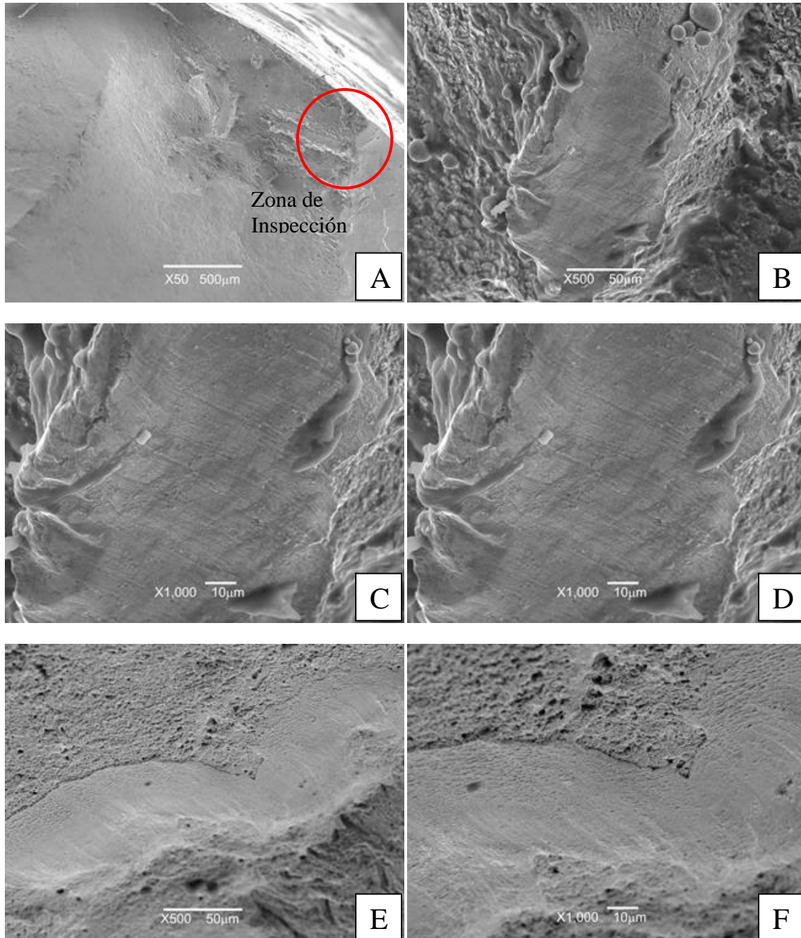
Figura 4.21 Fractografías del alambre EN-20110401-008-C1
