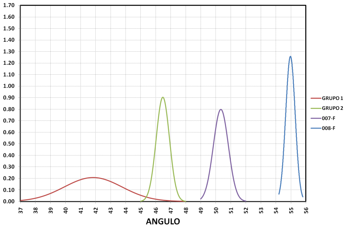
Figura 4.16 Comparativa del ángulo de ruptura por falla diagonal
