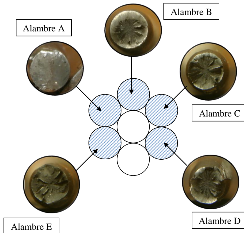
Figura 4.9 Identificación de las rupturas de los alambres del torón EN-20110401-001
