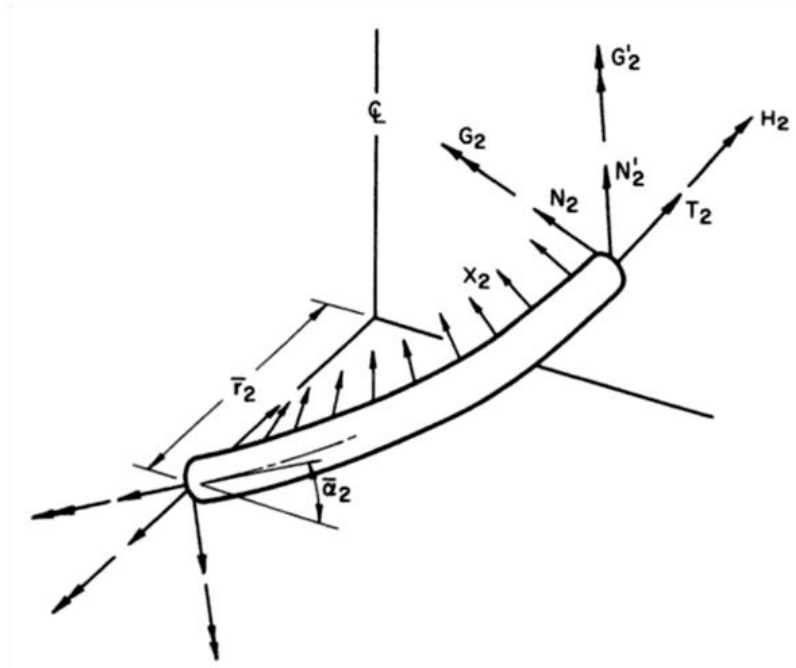
Figura 2.25 Fuerzas que actúan en un alambre helicoidal
