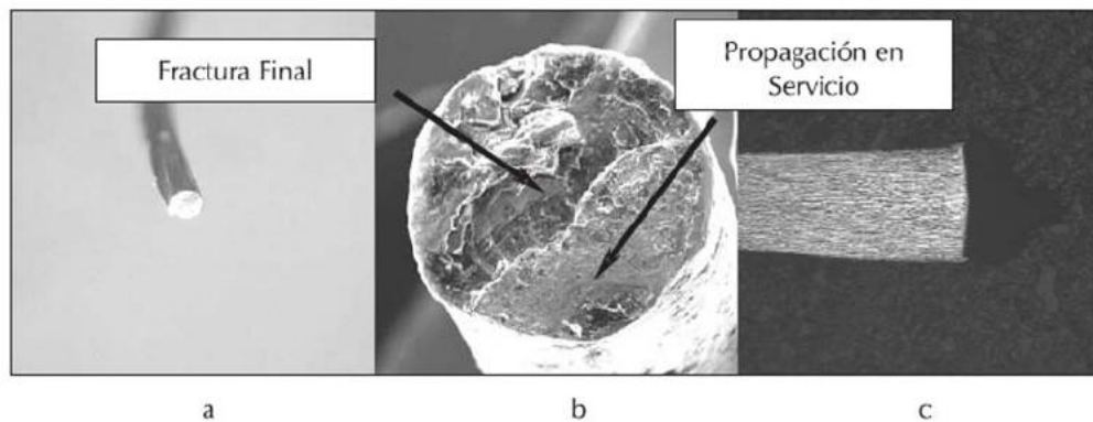
Figura 7. Fractura típica por fatiga en un alambre de un torón de presfuerzo. [2] a) Fractura por fatiga plana y perpendicular al eje b) Superficie de fractura perpendicular al eje del alambre, c) Granos sin deformación plástica en el alambre con fractura por fatiga perpendicular al eje
