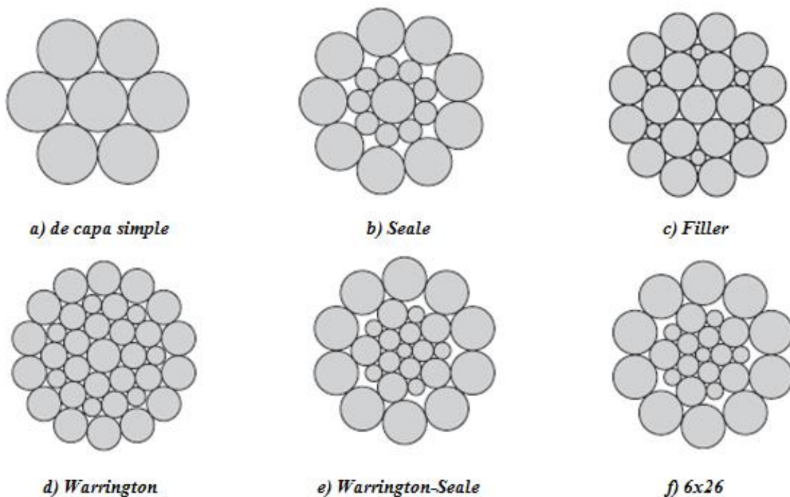
Figura 2.17 Construcciones comunes de torones Fuente: Manual Union, y Manual Emcables, 2008.
