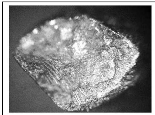
Figura 2.21 Estriaciones formadas por fatiga en un alambre de un torón
