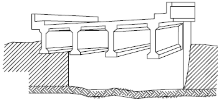
Figura 2.8 Puente losa con traves pretensadas Fuente: Dirección General de Caminos y Ferrocarriles, 2006.
