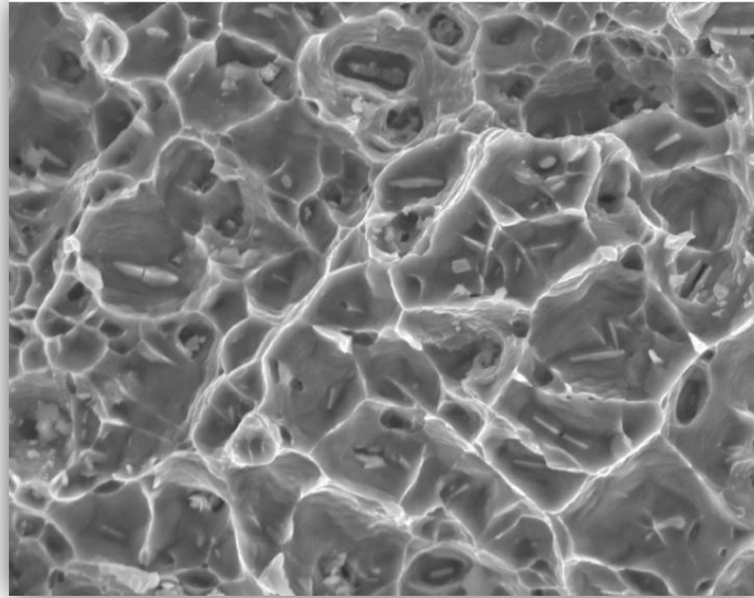
Figura 2.31 Cavidades o Dimples
