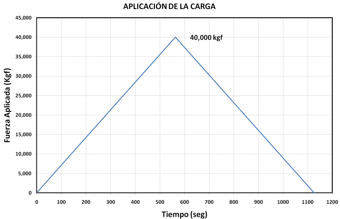
Figura 3.8 Curva de aplicación de carga.
