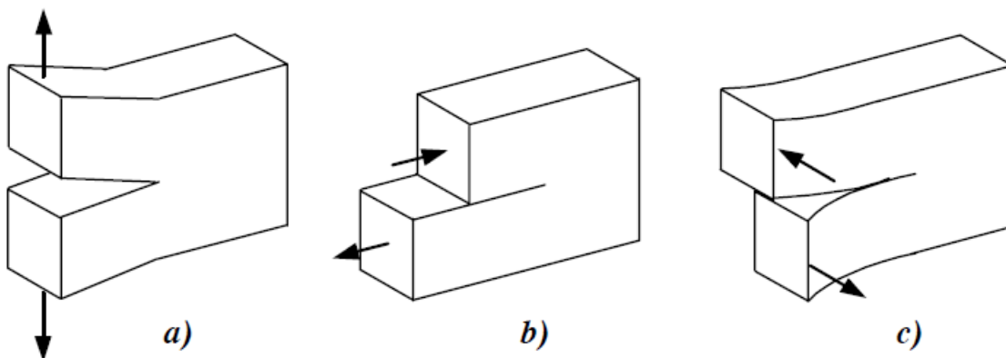
Figura 2.26 Diferentes Modos de carga, a) Modo I en tensión, b) Modo II en cortante y c) Modo III en desgarramiento.
