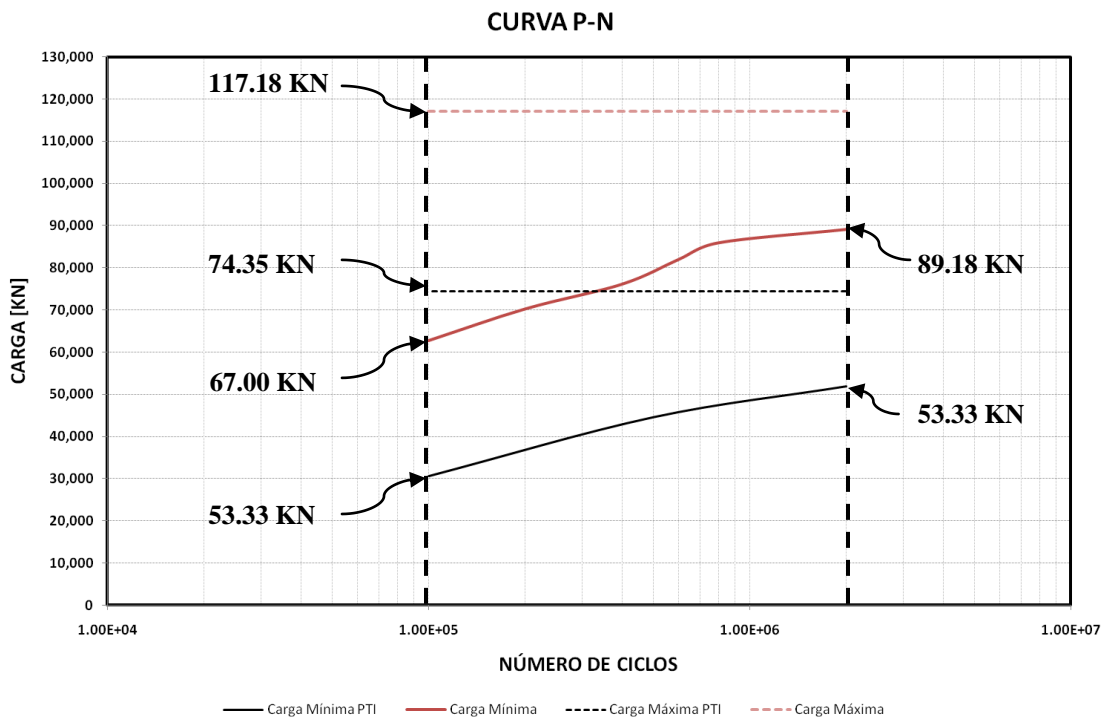
Figura 3.4 Carga contra número de ciclos propuesta para las pruebas.
