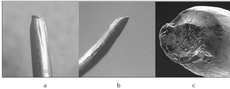
Figura 6. Fracturas en servicio por sobrecarga en torones de presfuerzo. [2] a) Alambre con formación de cuello y fractura tipo copa-cono, 7X b) Alambre con formación de cuello y fractura a 45° aproximadamente, 7X c) Alambre con formación de cuello y fractura tipo copa-cono, SEM 33X
