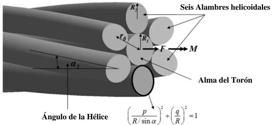
Figura 2.22 Topología de un torón de capa simple
