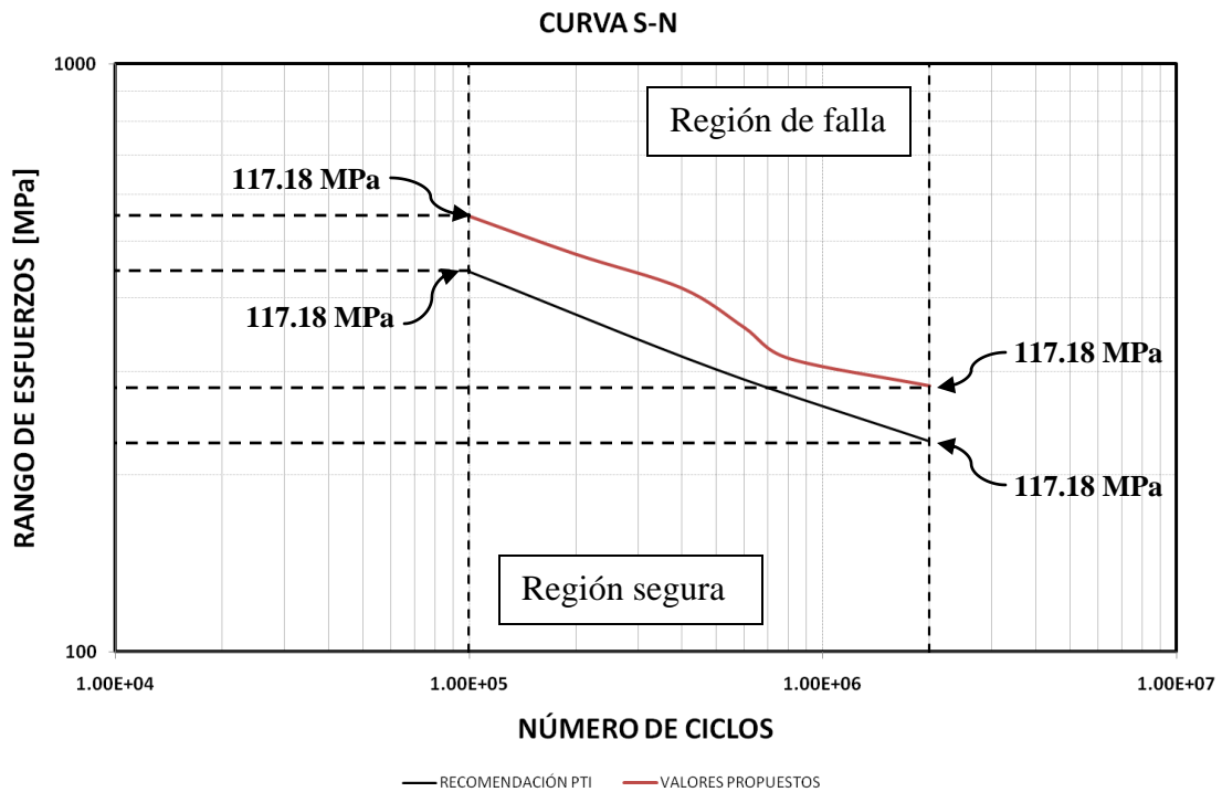
Figura 3.3 Curva propuesta para las pruebas de fatiga.
