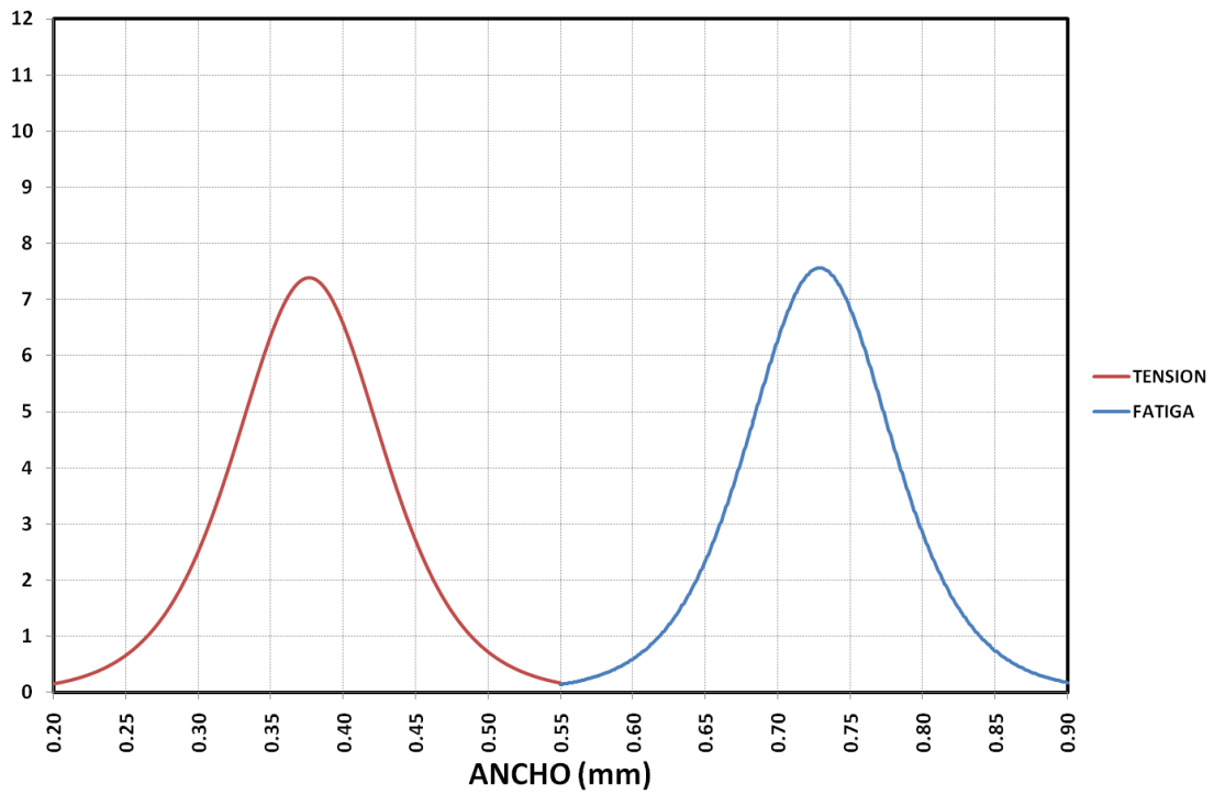
Figura 4.17 Comparativa del daño causado por la incrustación de la mordaza a lo ancho
