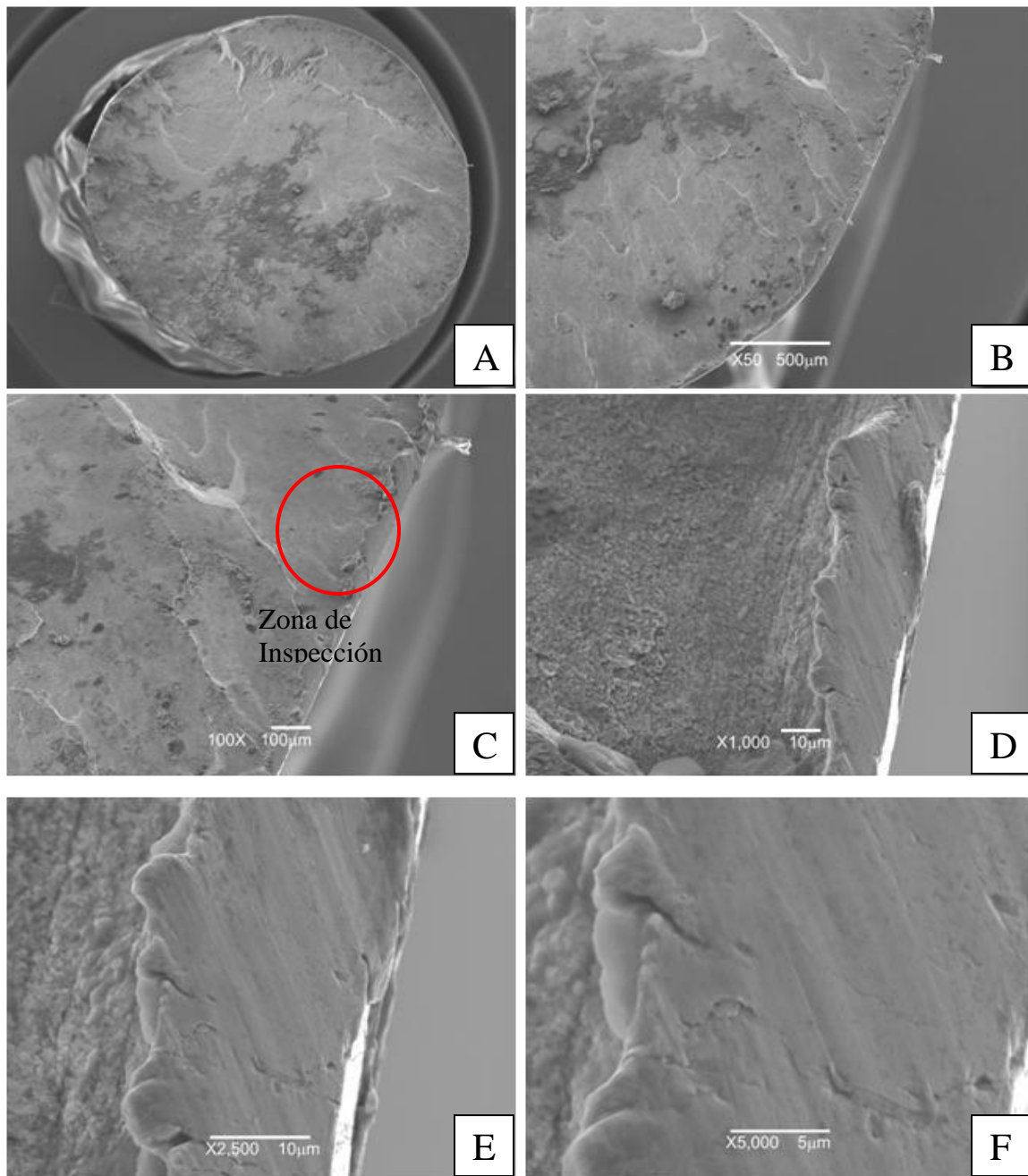
Figura 4.24 Fractografías del alambre EN-20110401-008-F2
