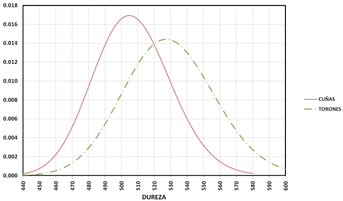
Figura 4.8 Comparativa de distribuciones de dureza entre el torón y las cuñas de anclaje
