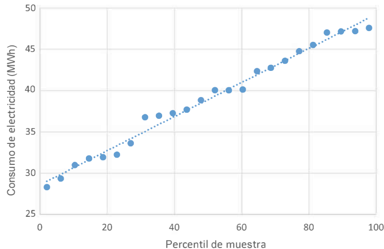
Figura 6.17: Indicador de desempeño energético (2018-2019).
