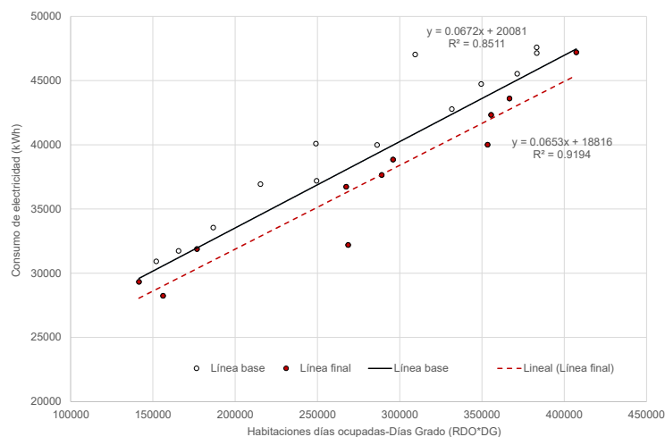
Figura 6.14: Línea base y línea objetivo de consumo de energía vs HDO*DG (2018-2019).
