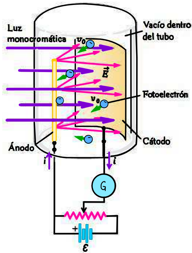
Figura 2.1: Experimento sobre el efecto fotoeléctrico desarrollado por los científicos alemanes Philipp Lenard y Wilhelm Hallwachs entre 1886 y 1900.
