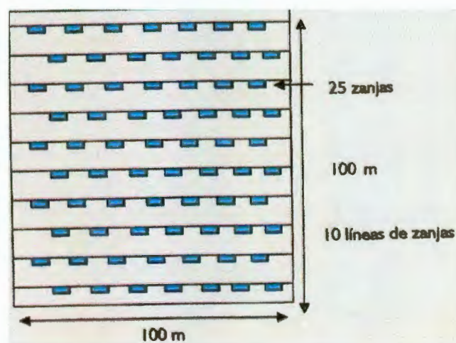
Figura. 49. Distribución de zanjas trincheras en una hectárea.
