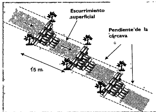
Figura. 31. Distribución espacial de presas de costales en una cárcava.
