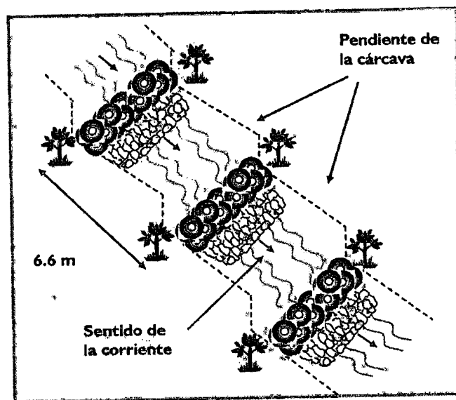
Figura. 33. Distribución espacial de presas de llantas en una cárcava.
