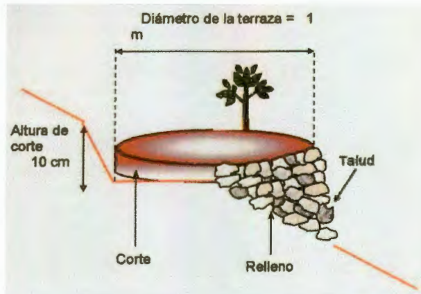
Figura.45. Dimensiones de terraza individual.
