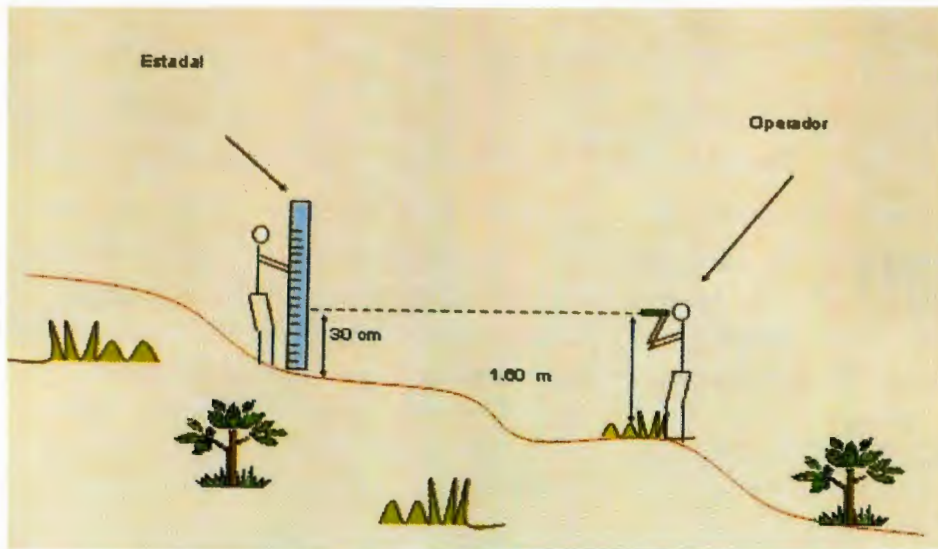
Figura.10. Determinación de pendiente con nivel de mano.
