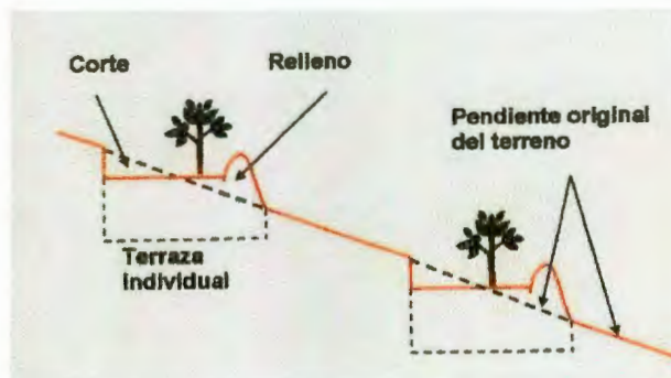
Figura. 44. Sección transversal de terrazas individuales.
