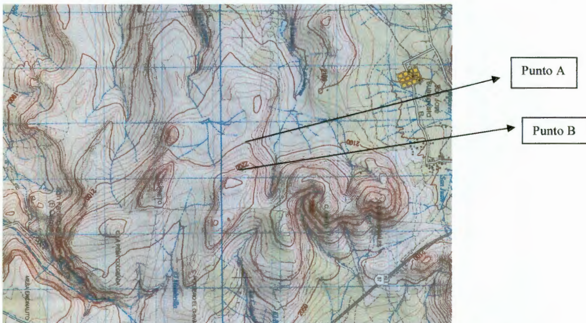
Figura.11. Determinación de pendiente con una carta topográfica.
