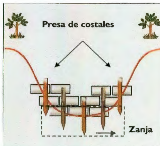
Figura. 29. Colocación de estacas en presas de costales.
