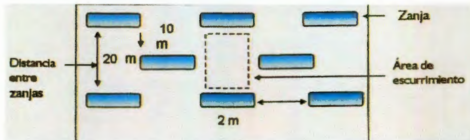
Figura.48. Diagrama de distribución de tinajas ciegas en tresbolillo.
