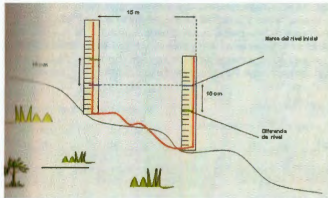
Figura.9. Medición de pendiente con nivel de manguera.
