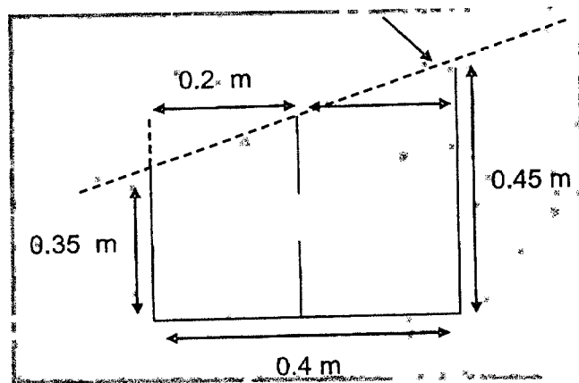
Figura. 47. Sección transversal del diseño de una presa en terreno con pendiente.
