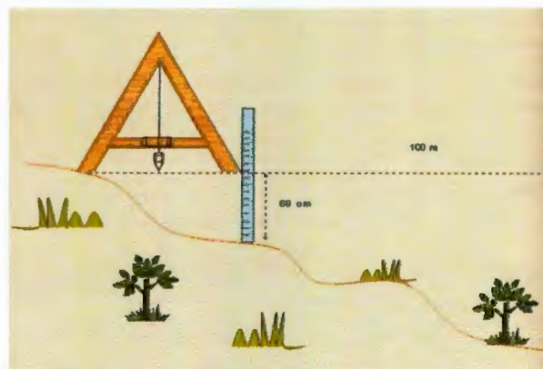
Figura. 8. Medición de la pendiente con el aparato "A"
