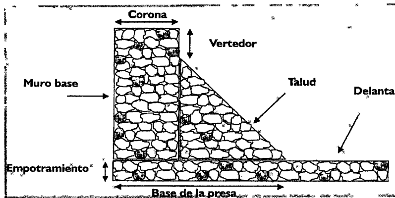
Figura. 26. Partes que constituyen a una presa de piedra acomodada.
