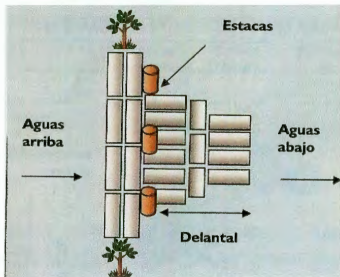
Figura. 30. Diseño de presa de costales con delantal. (Vista horizontal).
