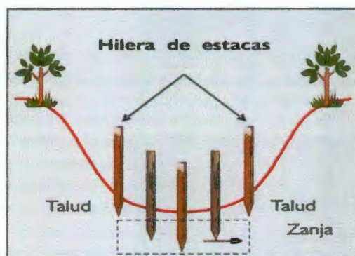
Figura.19. Colocación transversal de hilera de estacas.
