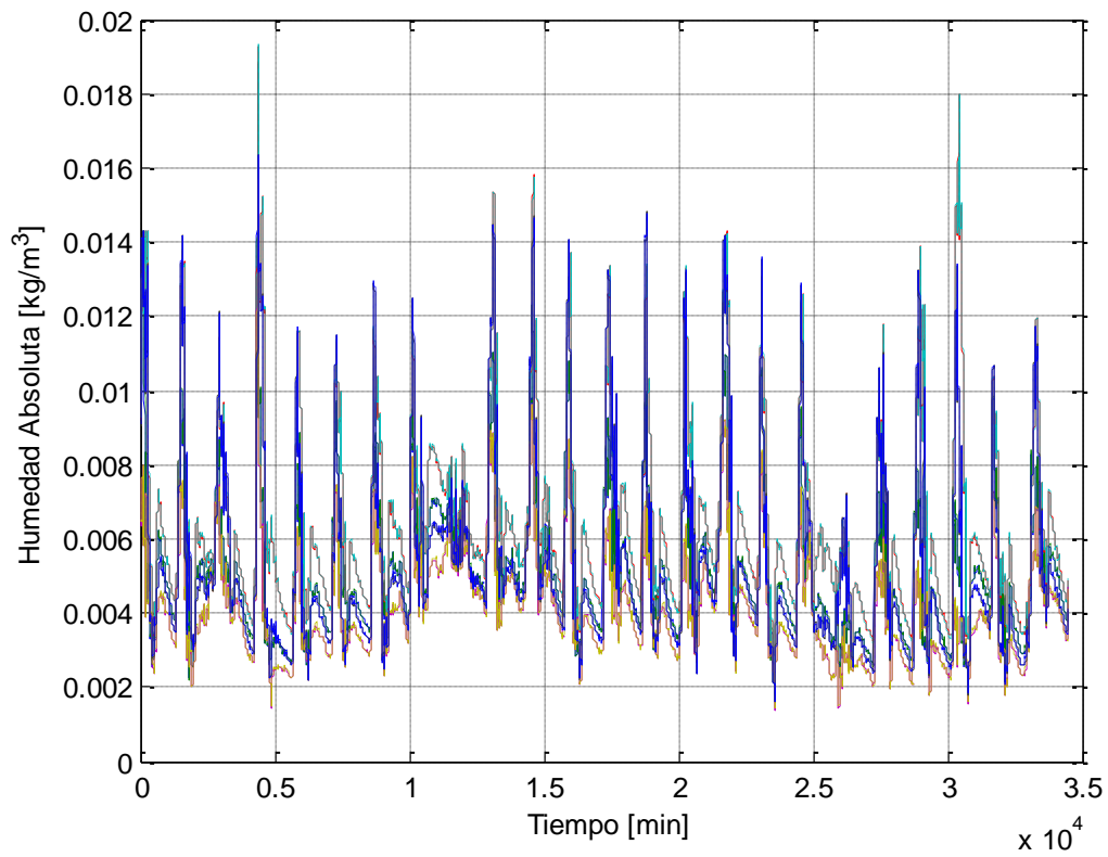
Figura 4.16 Datos medidos y datos estimados correspondientes a la humedad absoluta en la segunda corrida (del 4 al 29 de Diciembre de 2012).
