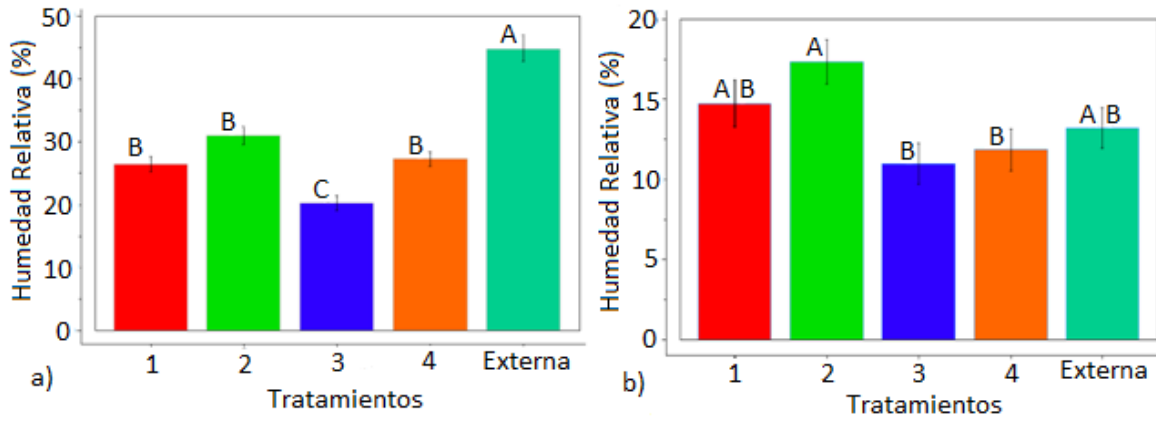
Figura 4.4 Comparación de medias de humedad relativa mínima en los cuatro tratamientos y el exterior a un nivel de significancia de P \leq 0.05 . a) Sep.-Oct. y b) Diciembre.
