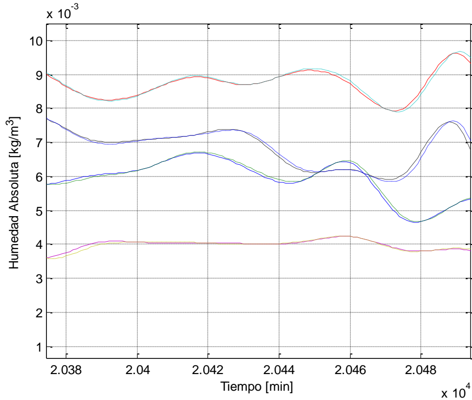
Figura 4.17 Ampliación de los datos medidos (—) y datos estimados (- -) correspondientes a la humedad absoluta en la segunda corrida (del 4 al 29 de Diciembre de 2012).
