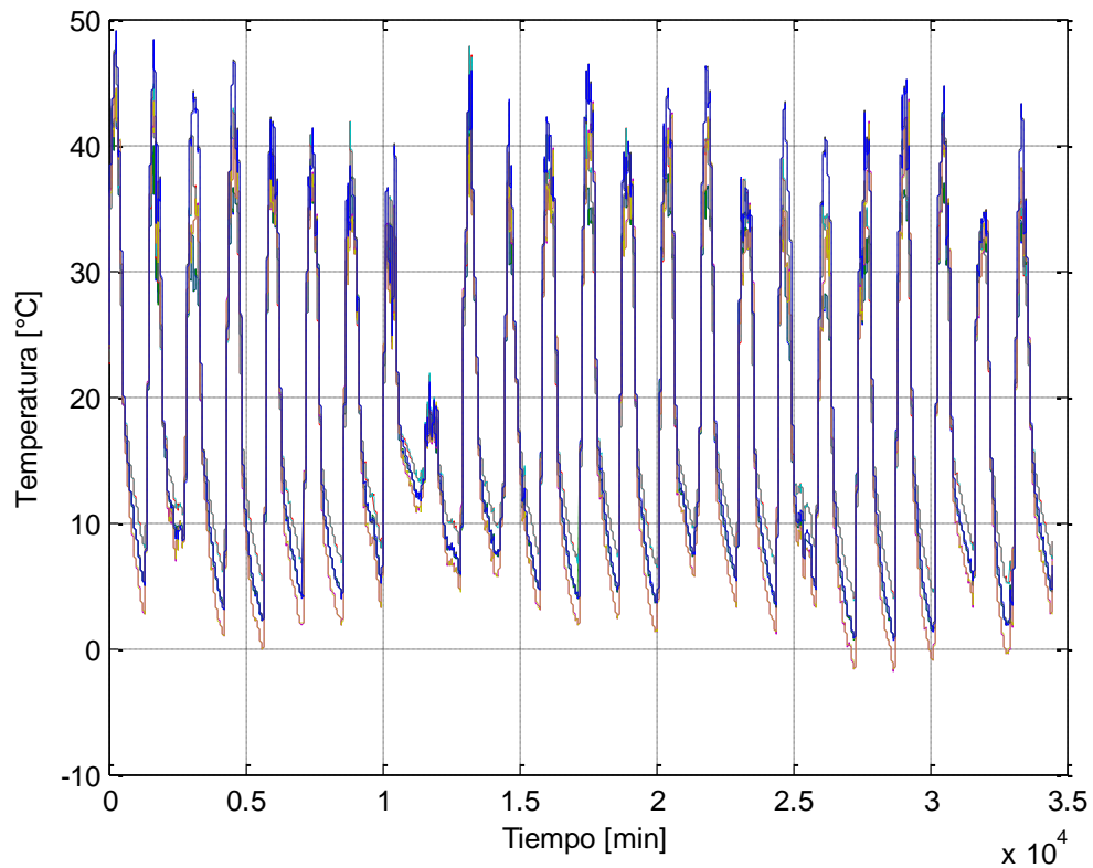
Figura 4.14 Datos medidos y datos estimados correspondientes a la temperatura en la segunda corrida (del 4 al 29 de Diciembre de 2012).
