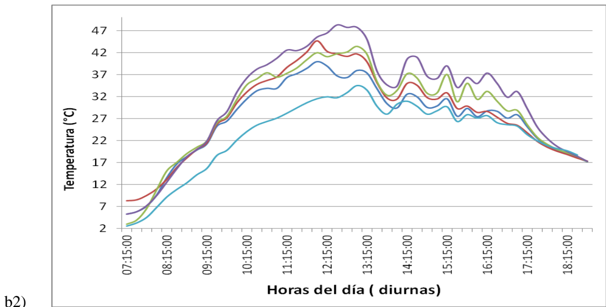
Figura 4.1 Temperaturas de un día del cultivo a1) y a2) 12 de Septiembre de 2012 y b1) y b2) 4 de Diciembre de 2012.
