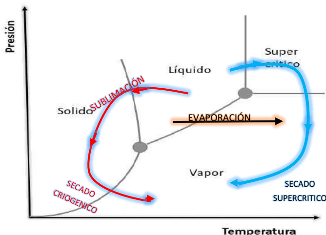
Fig. 2.3 Diagrama de fases de un fluido y esquematización de los tres tipos de secado posibles en la síntesis de aerogeles.
