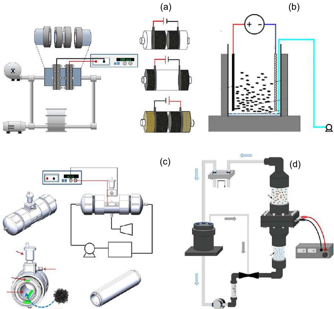
Figura 9. Reactores con configuración tridimensional de diferentes estudios. (a) Reactor electro-Fenton cilíndrico (Flow-trough) con electrodos de fieltro de grafito y resinas con Fe(II), (b) diagrama de la reacción electroquímica 3D fluidizado, (c) reactor electro-Fenton cilíndrico con electrodos de carbón poroso y carbón activado y (d) reactor electro-Fenton heterogéneo fluidizado a escala piloto (García-Espinoza et al. , 2021; Liu et al. , 2022; García-Espinoza et al. , 2021 y Poza-Nogueira et al. , 2021, respectivamente).
