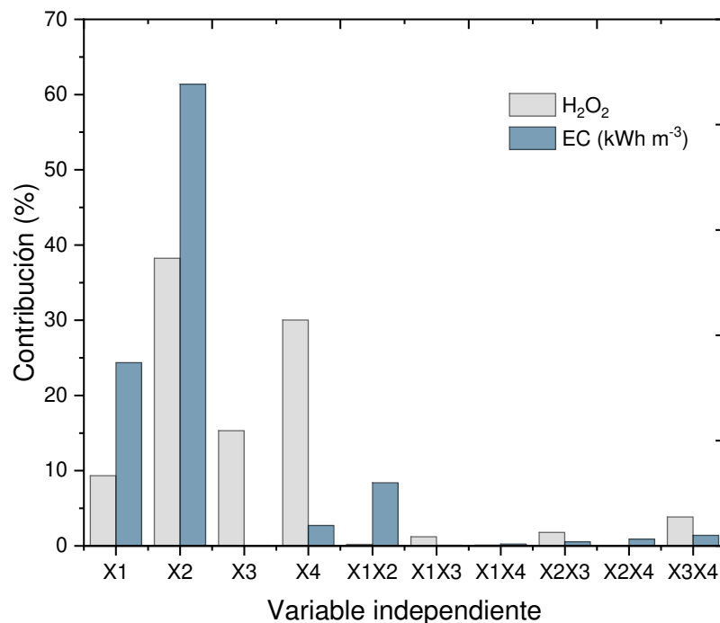
Figura 19. Análisis gráfico de Pareto sobre el efecto del tiempo (min)- X_1 , densidad de corriente ( mA\ cm^{-2} )- X_2 , fuerza iónica (mM)- X_3 y configuración experimental- X_4 , en la generación del H_2O_2 y el consumo energético.
