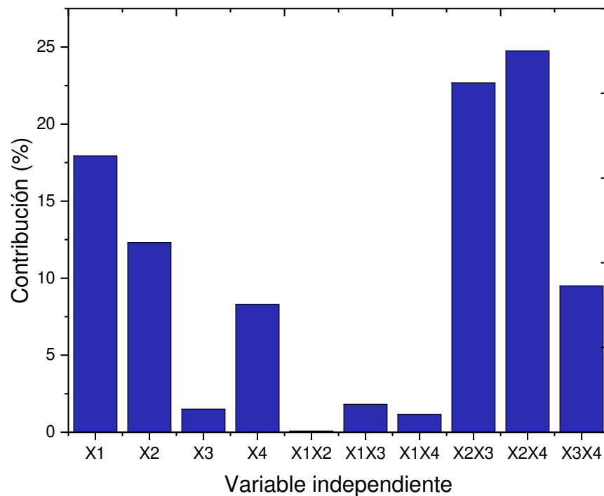
Figura 22. Análisis gráfico de Pareto sobre el efecto del tiempo (min)- X_1 , cantidad de resina Fe(II) (g)- X_2 , cantidad de CAG (g)- X_3 y radiación UV- X_4 , en la degradación de la CBZ.
