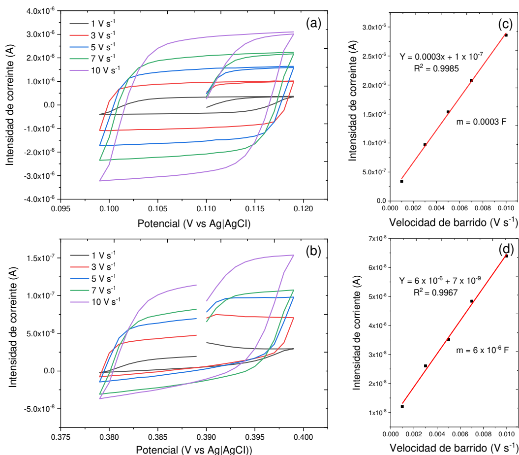
Figura 16. Voltamperogramas cíclicos del área electroactiva: (a) fieltro de grafito, (b) CAG, (c) y (d) regresión lineal del fieltro de grafito y el CAG respectivamente.
