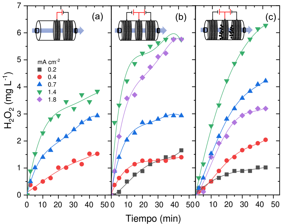
Figura 18. Concentración de H 2 O 2 a diferentes densidades de corriente. (a) ánodo-cátodo, (b) cátodo-ánodo-cátodo y (c) cátodo-ánodo-cátodo CAG. [Na 2 SO 4 ] 0.05 M, pH 0 = 7, Q = 7 L min -1 .
