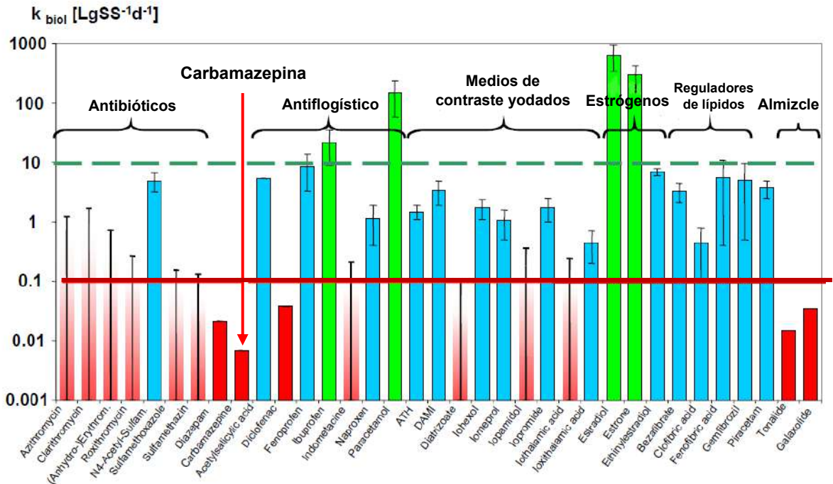
Figura 4. Constantes de velocidad de degradación biológica de pseudo primer orden k_{biol} observadas en experimentos aeróbicos por lotes realizados con lodos activados de PTAR con una edad de lodos \geq 8 d. Línea roja en k_{biol} 0.1 \text{ L gSS}^{-1} \text{ d}^{-1} indica el límite por debajo del cual no se espera degradación significativa en las PTAR municipales (Joss et al. , 2005).
