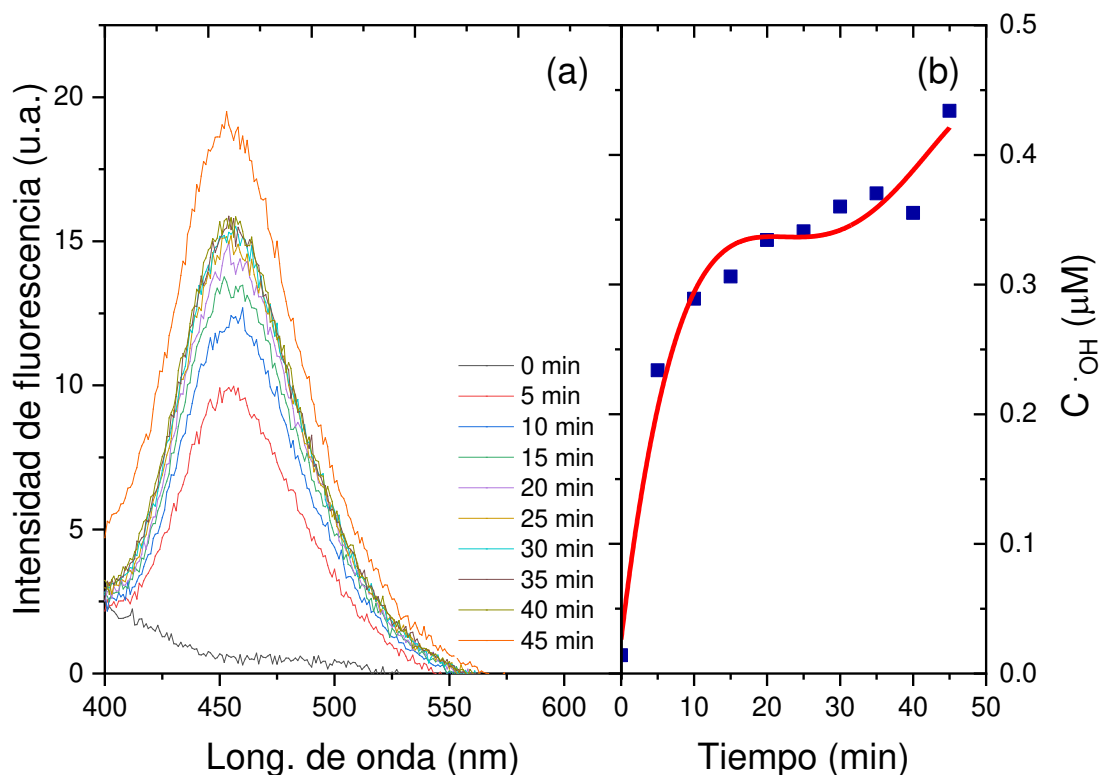
Figura 21. (a) Espectro de fluorescencia de la 7-HC y (b) C_{\cdot\text{OH}} ( \mu\text{M} ).
