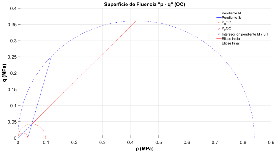
Figura 4-26 Superficie de fluencia con un grado de preconsolidación \lambda = 24
