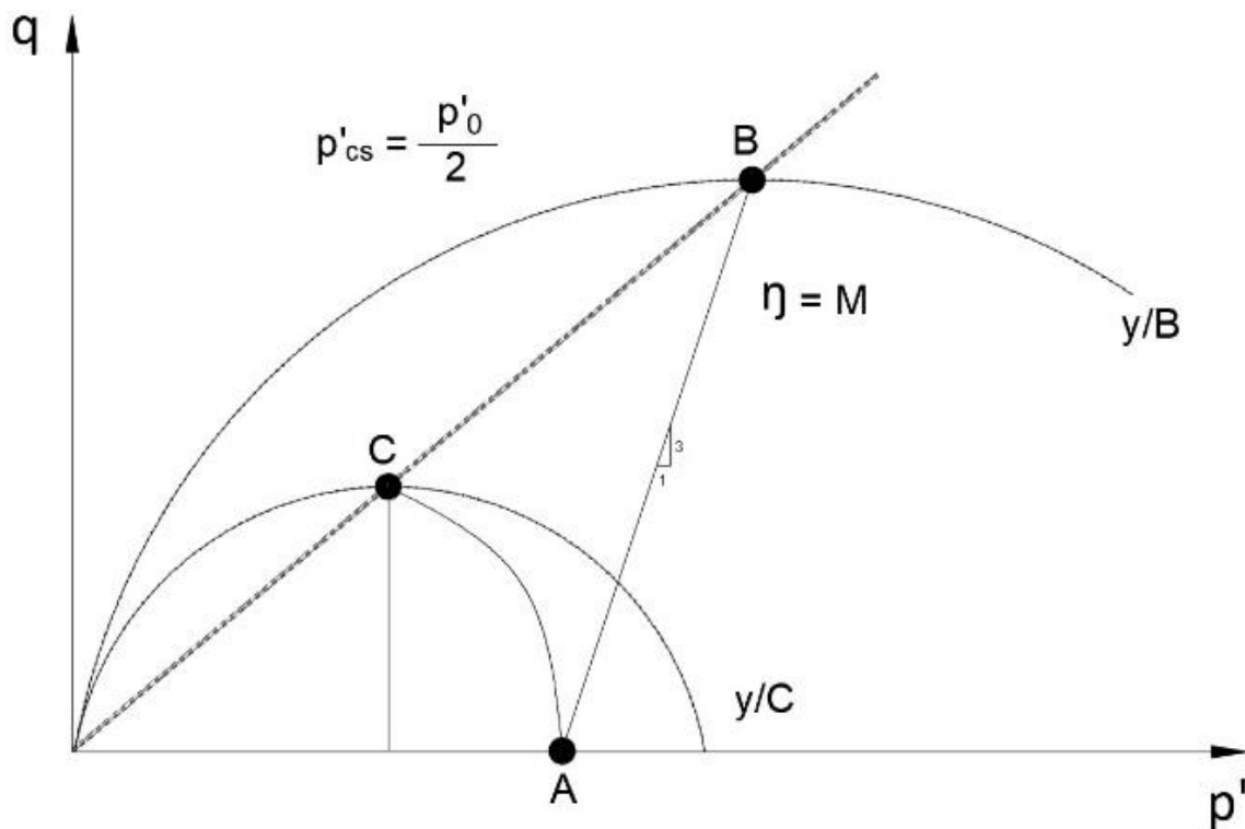
Figura 2-8 Ensaye triaxial drenado (AB) y no drenado (AC) para muestras normalmente consolidadas y ligeramente preconsolidados.
