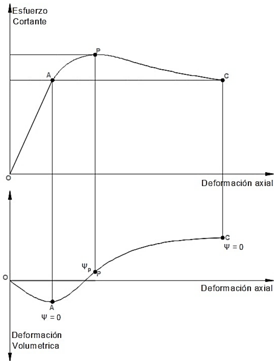
Figura 2-2 Esfuerzo, deformación cortante y dilatación en una prueba triaxial (Atkinson,1993)
