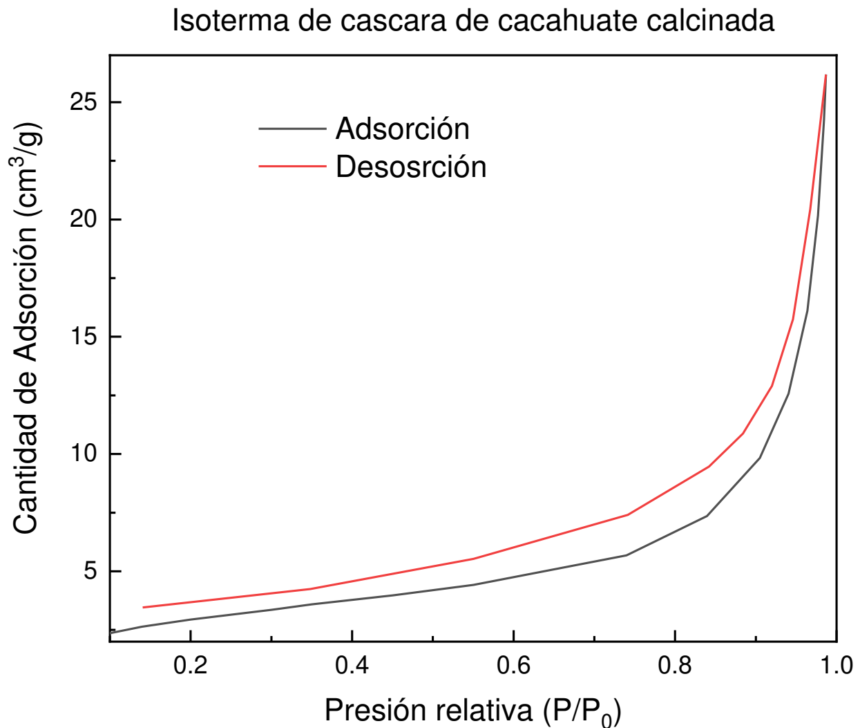
Figura 26 Isooterma de adsorción de cascara de cacahuate calcinada
