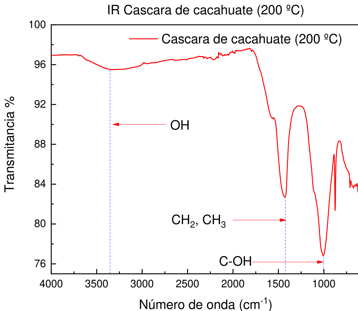
Figura 14 IR de cascara de cacahuate calcinada a 200 °C
