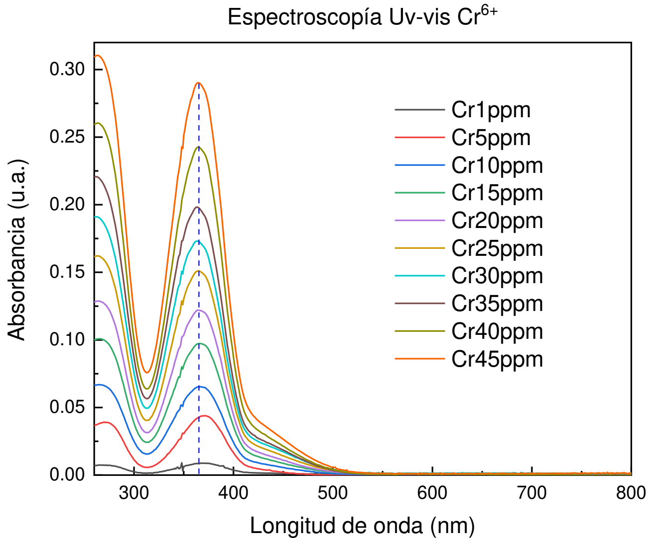
Figura 18 Espectroscopia Uv-vis obtenida de alícuotas de diferente concentración de Cromo hexavalente
