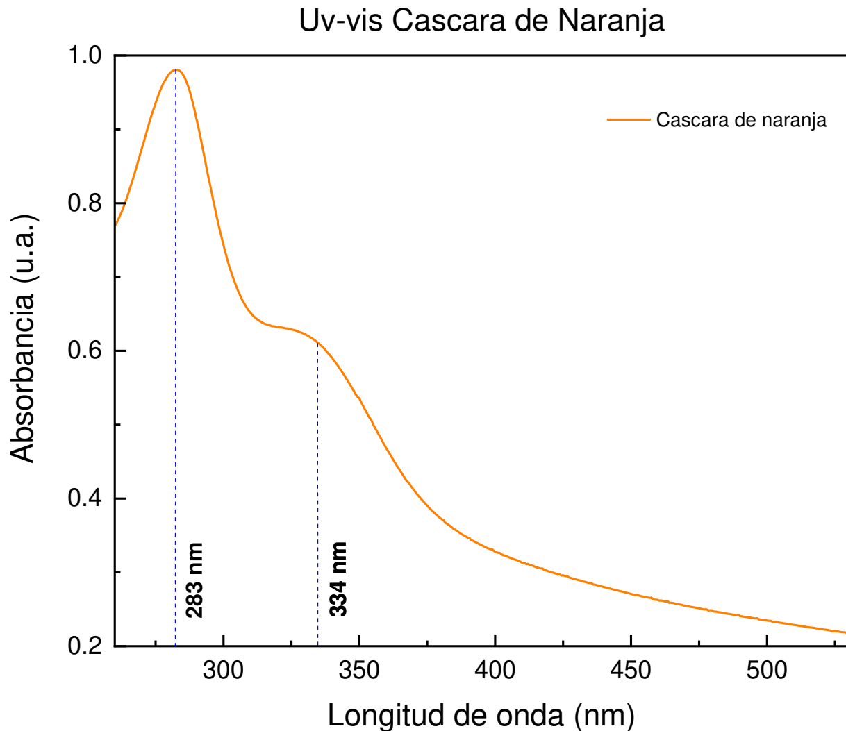
Figura 16 Análisis espectrofotométrico ultravioleta-visible de cascara de naranja
