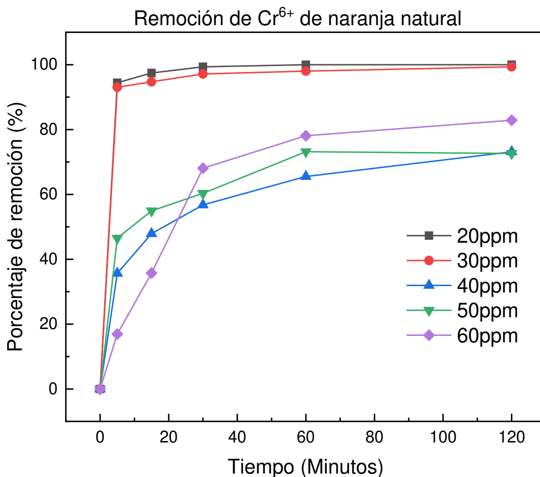
Figura 20 Cinética de remoción de cromo hexavalente de cascara de naranja natural
