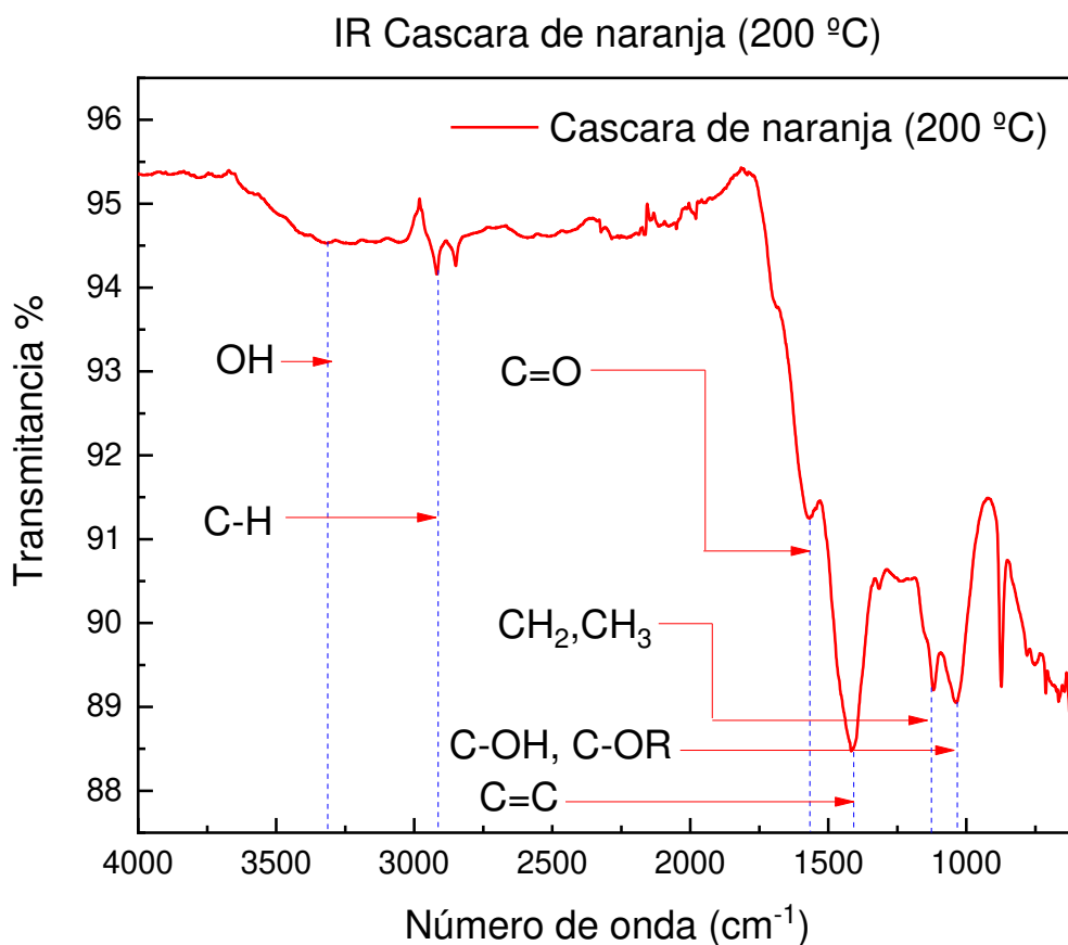
Figura 11 IR de cascara de naranja calcinada a 200 °C
