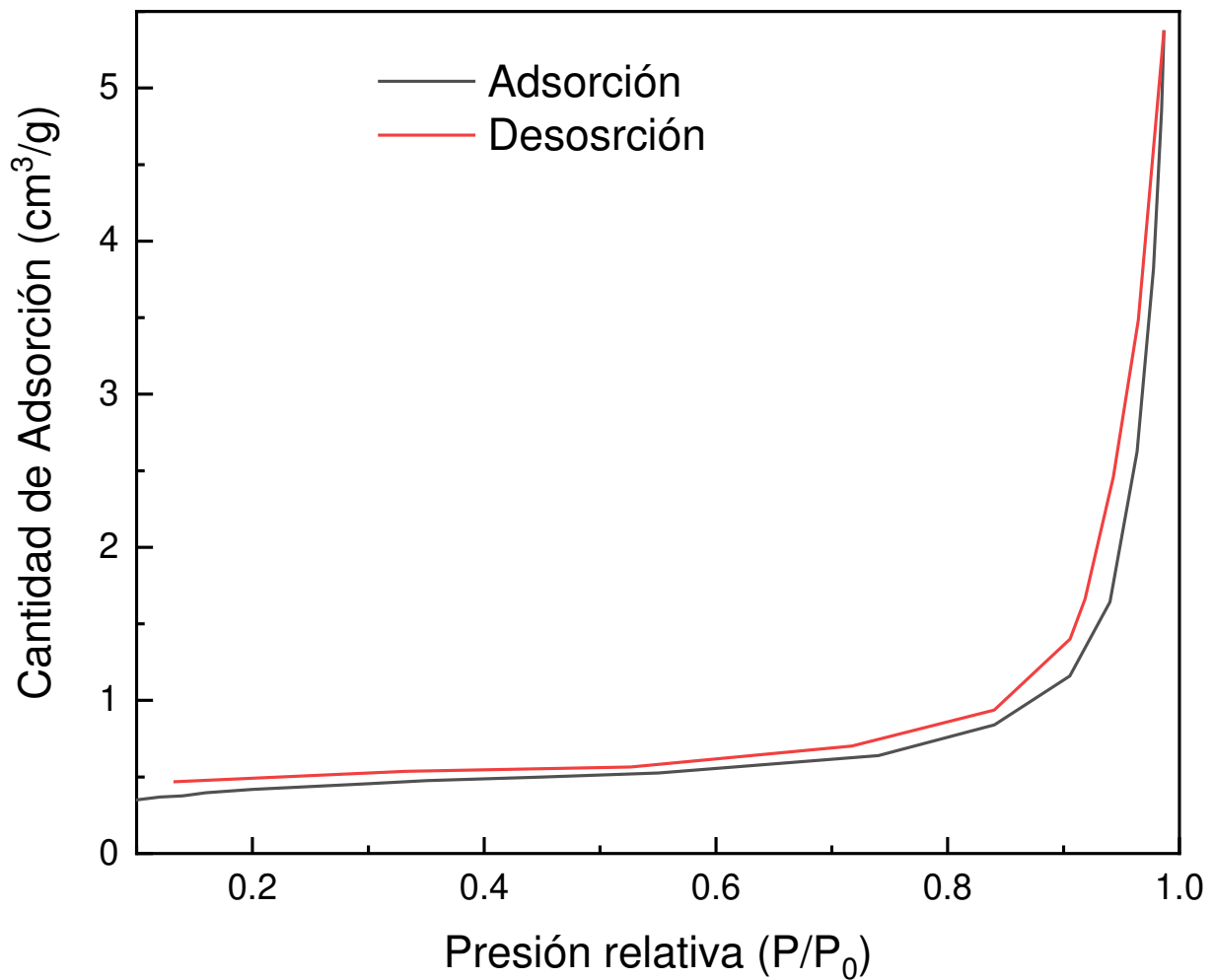
Figura 25 Isoterma de adsorción de cascara de naranja calcinada
