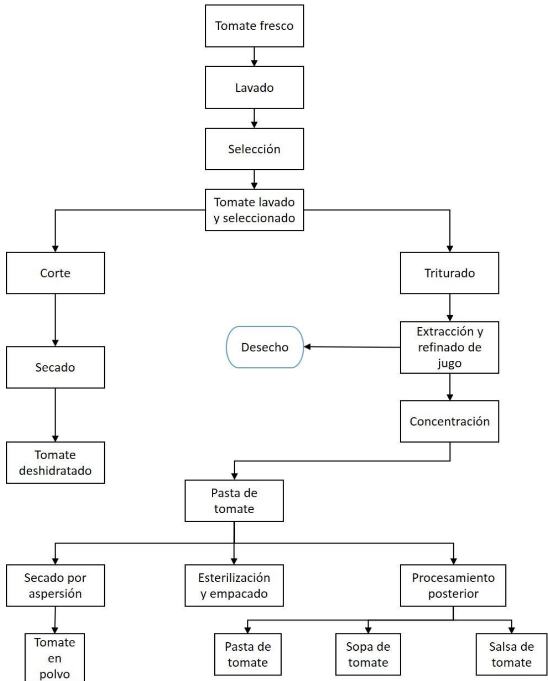
Anexo I-B. Diagrama general de procesamiento de jitomate. (Hui et al., 2004).
