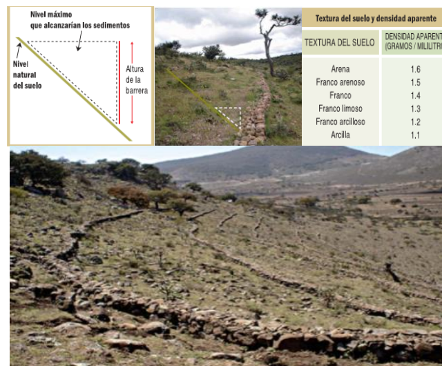
Figura 23. Barreras de piedra acomodada en curvas de nivel.
