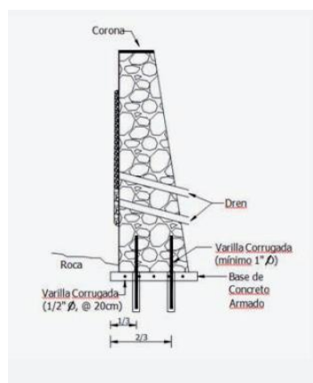
Figura 21. Muro de contención de mampostería.
