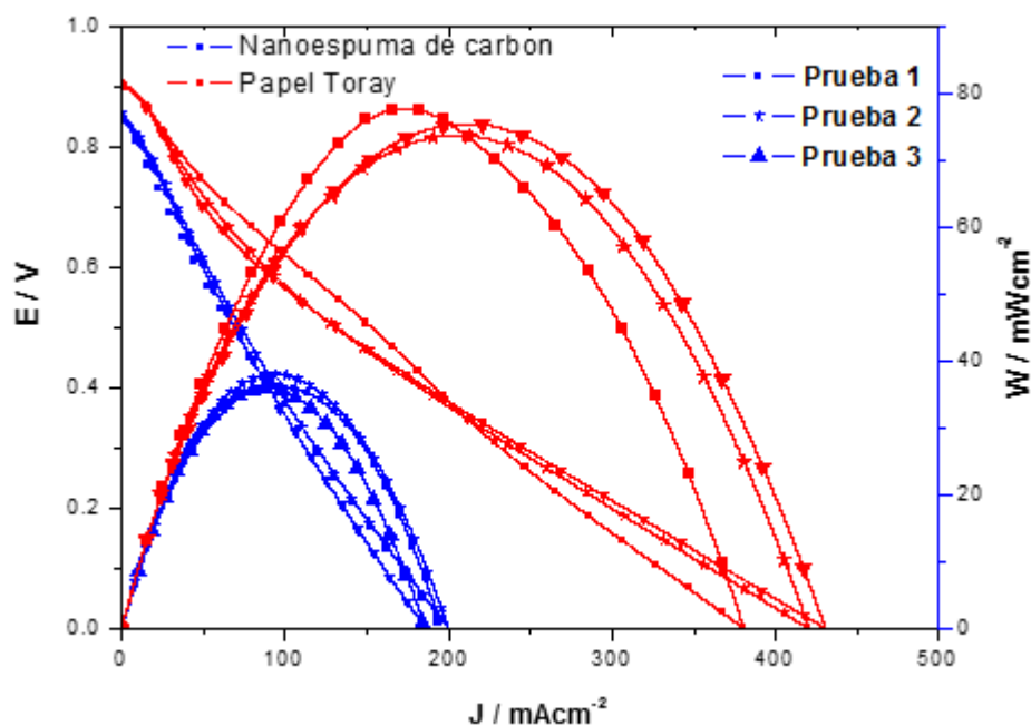
Figura 16.-Curvas de polarización y de densidad de potencia después de tres pruebas con combustible de ácido fórmico ( \text{HCOOH} ,) 1.5M flujo de 6 ml / h a temperatura ambiente de 25 °C para nanoespuma de carbón (azul) y papel Toray (rojo).
