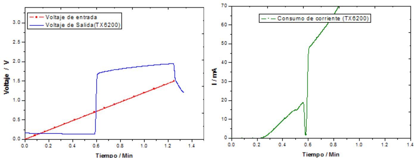
Figura 24.- Evaluación de circuito TPS61200
