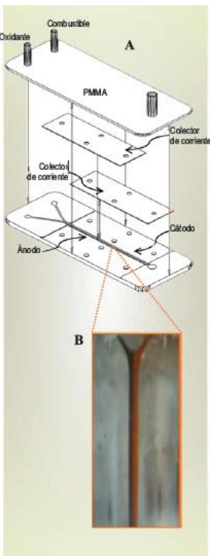
Figura 3.-A) Diagrama de ensamblaje de la celda de combustible basada en micro-fluidos laminares, construida en el CIDETEQ. B) Esquema del transporte laminar de los micro-fluidos
