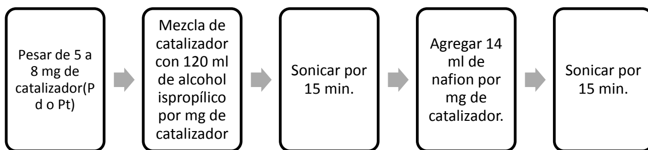
Figura 8.- Diagrama de elaboración de tintas catalíticas
