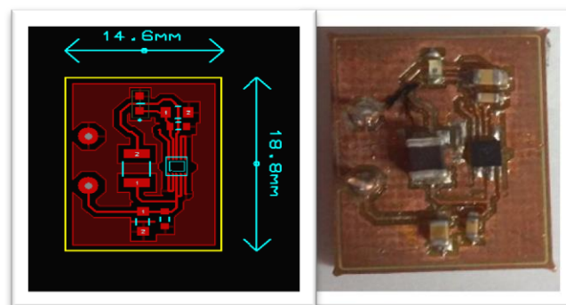
Figura 21.- Miniaturización de circuito TS3310
