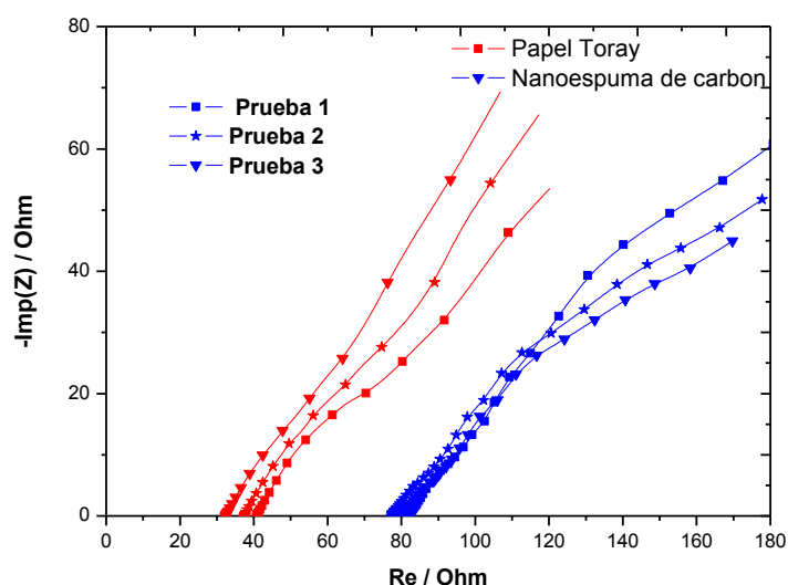
Figura 17.- Impedancias de tres pruebas con combustible de ácido fórmico ( \text{HCOOH} ), 1.5M flujo de 6 ml / h a temperatura ambiente de 25\ ^\circ\text{C} para nanoespuma de carbón (azul) y papel Toray (rojo).
