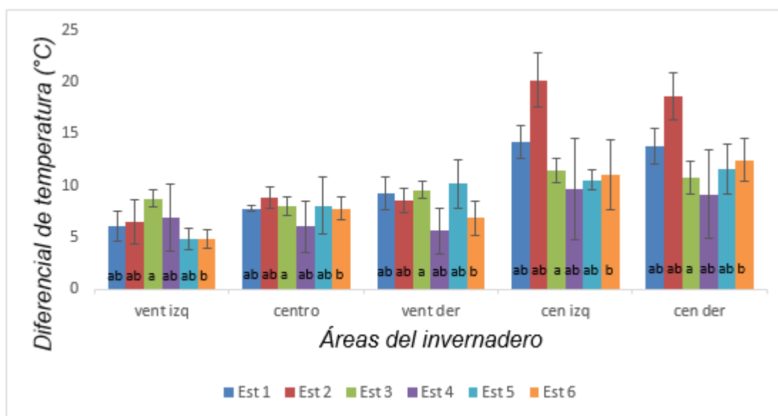
Figura 6.6 Diferencial de temperatura del promedio de 11 am a 3 pm entre las diferentes estrategias en las diferentes partes del invernadero.
