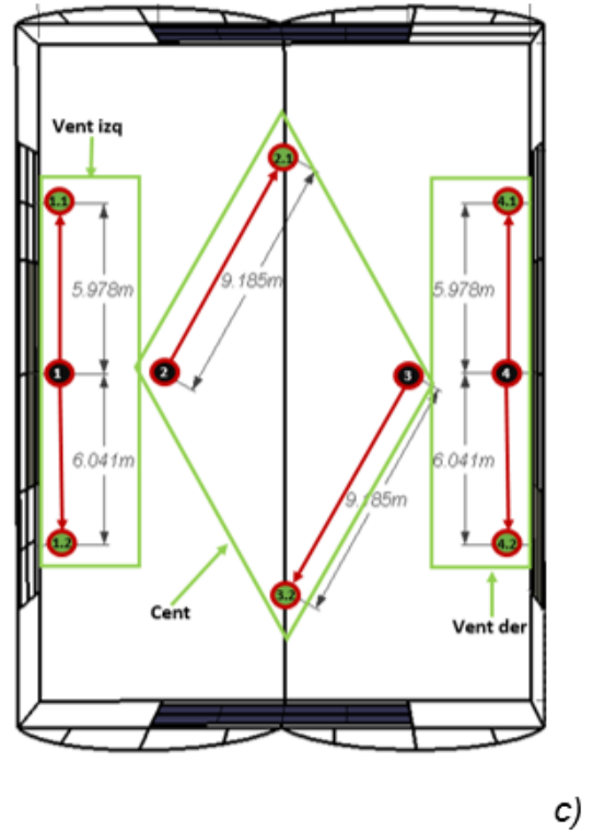
Figura 5.4 Distribución de sensores dentro del invernadero. Los círculos marcados como negro y rojo son los dataloggers y los marcados con verde y rojo son los sensores que están conectados al datalogger, las flechas indican que sensor de temperatura está conectado al datalogger a) vista frontal de sensores de diferencial de altura (efecto invernadero) colocados en el centro de cada nave. b) sensores colocados a través de la
