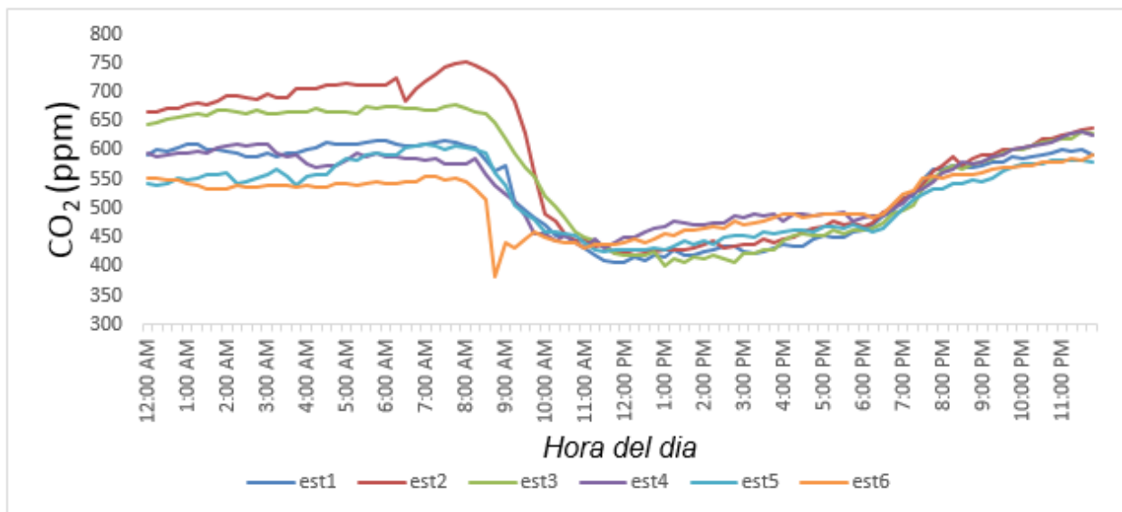
Figura 6.11 Comportamiento promedio día de CO_2 de las estrategias.
