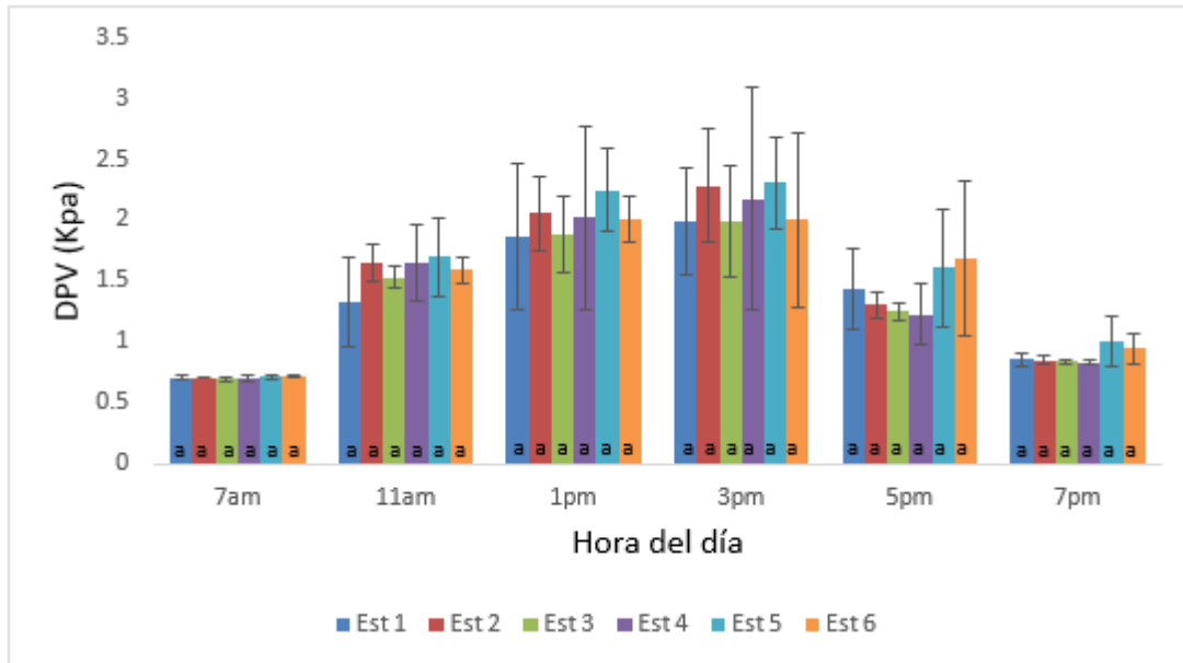
Figura 6.9 Déficit de presión de vapor de los diferentes puntos del invernadero con las diferentes estrategias.
