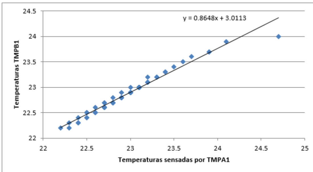
Figura 6.2 Caracterización del sensor de temperatura TMPB1 sobre TMPA1.
