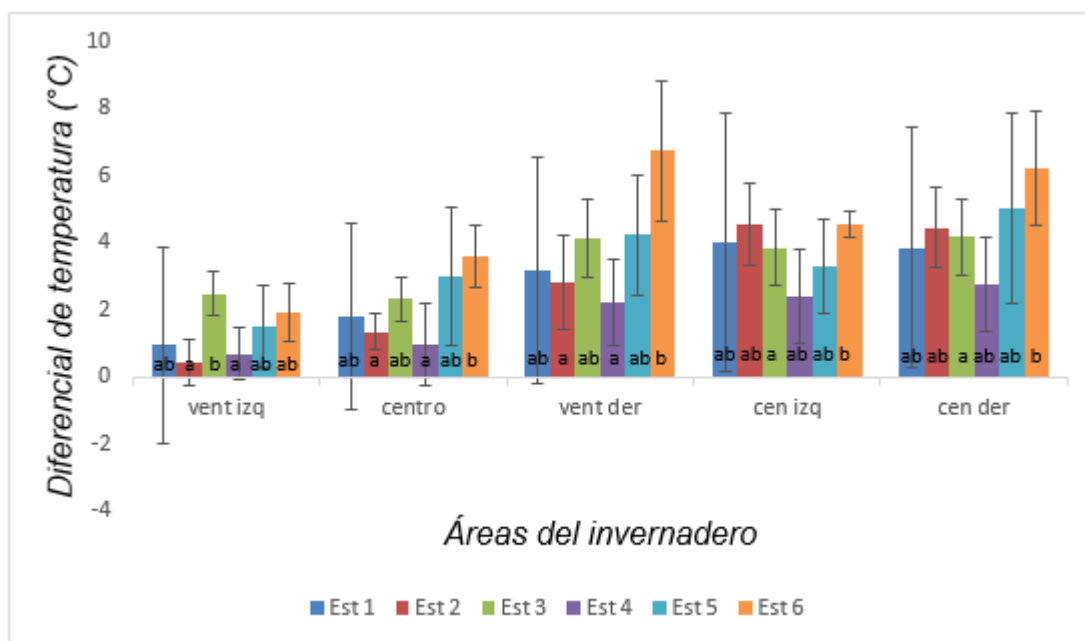
Figura 6.7 Diferencial de temperatura del promedio de 3 pm a 7 pm entre las diferentes estrategias en las diferentes partes del invernadero.
