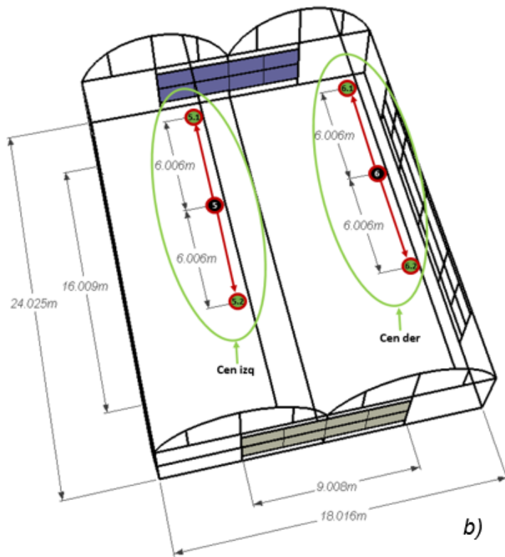
Figura 5.4 Distribución de sensores dentro del invernadero. Los círculos marcados como negro y rojo son los dataloggers y los marcados con verde y rojo son los sensores que están conectados al datalogger, las flechas indican que sensor de temperatura está conectado al datalogger a) vista frontal de sensores de diferencial de altura (efecto invernadero) colocados en el centro de cada nave. b) sensores colocados a través de la
