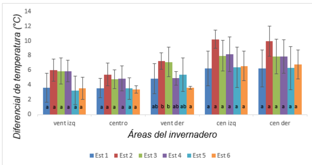
Figura 6.5 Diferencial de temperatura del promedio de 7 am a 11 am entre las diferentes estrategias en las diferentes partes del invernadero.
