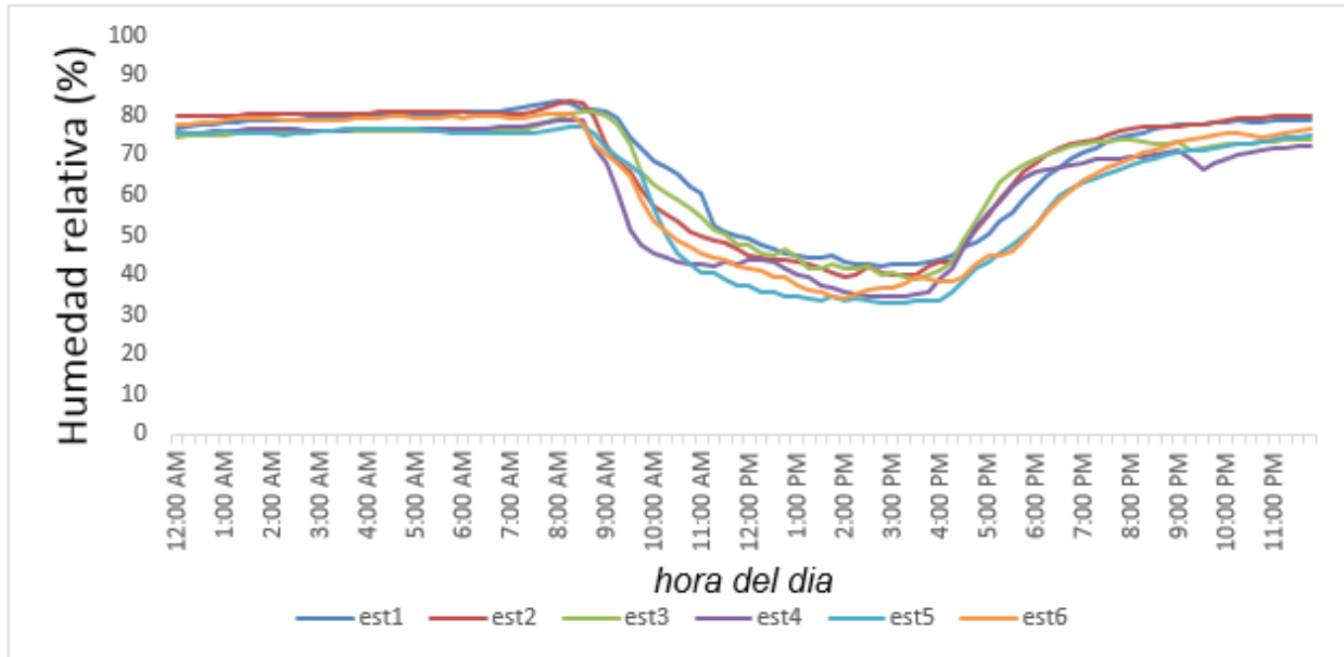
Figura 6.10 Comportamiento promedio día de HR de las estrategias.
