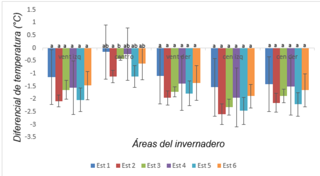
Figura 6.8 Diferencial de temperatura del promedio de 7 pm a 12 am entre las diferentes estrategias en las diferentes partes del invernadero.
