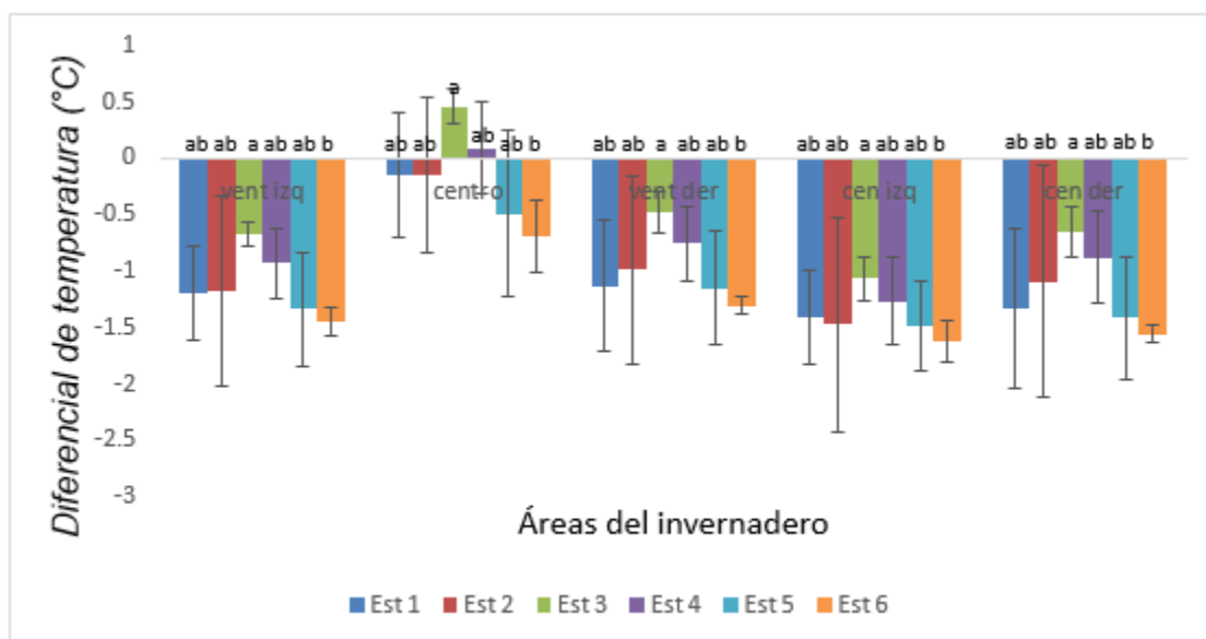
Figura 6.4 Diferencial de temperatura del promedio de 12 am a 7 am entre las diferentes estrategias en las diferentes partes del invernadero.
