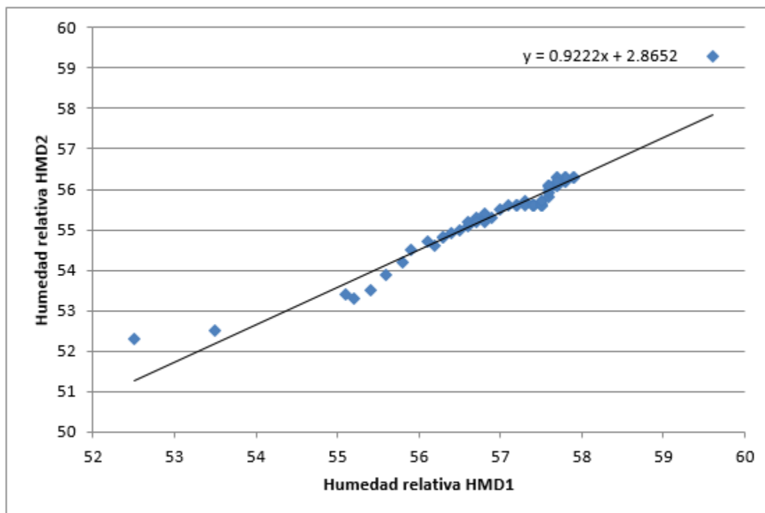
Figura 6.3 Caracterización del sensor de humedad relativa HMD2 sobre HMD1.
