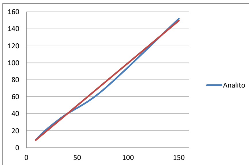
Figura 16. Curva de calibración del equipo Compact NO 3 - Meter TwinNO 3 - Modelo B-343, Marca HORIBA, Ltd.
