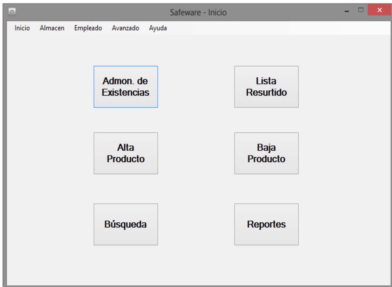
Figura 6-9 Pantalla Inicio
