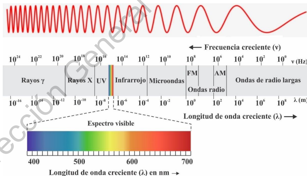
Figura 3. Espectro electromagnético
