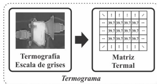
Figura 13. Matriz termal a partir de la imagen termográfica en escala de grises.
