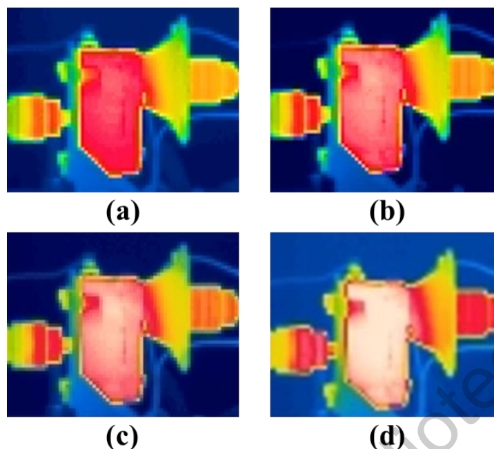
Figura 23. Imágenes termográficas para el monitoreo de la condición de engranajes en un sistema de transmisión de caja de engranajes: (a) HTL, y (b) 25%, (c) 50% y (d) 75% de desgaste uniforme en el engrane.
