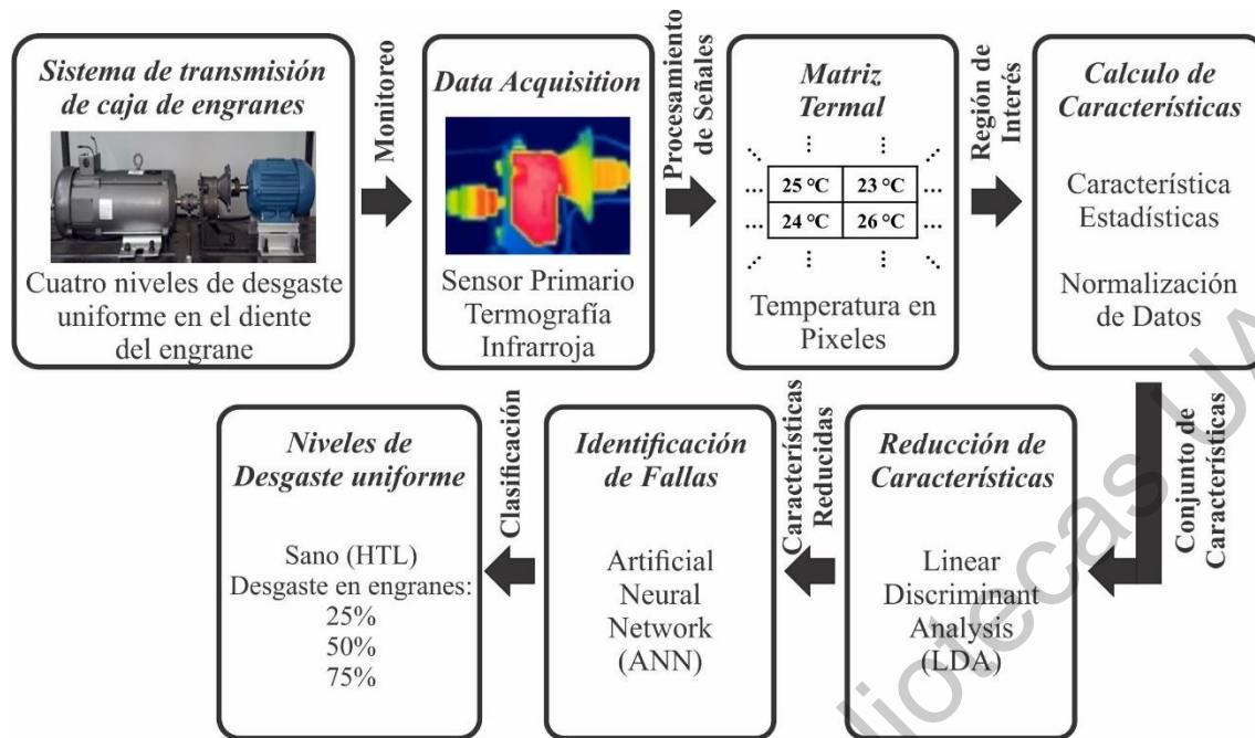
Figura 19. Metodología propuesta para identificar el desgaste uniforme del diente del engranaje de un sistema de transmisión de caja de engranajes.
