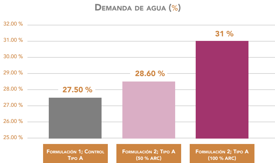
FIGURA 7. Resultados demanda de agua en % mezclas de adhesivos evaluados.
