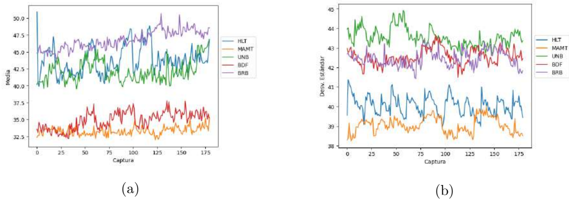
Figura 4.5: Evolución de indicadores termográficos en motor WEG: a) Media, b) Desviación Estándar
