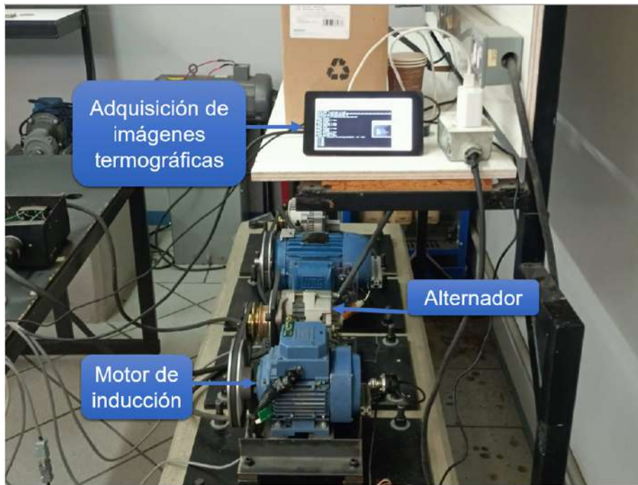
Figura 3.8: Banco de pruebas con motor de inducción trifásico WEG conectado a alternador mediante banda de transmisión
