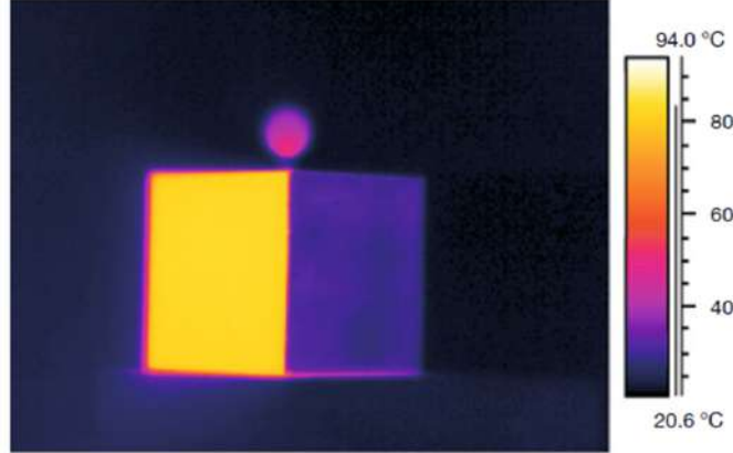
Figura 2.4: Termograma infrarrojo de un cubo de cobre con paleta de colores aplicada (Vollmer y Moellmann, 2018)
