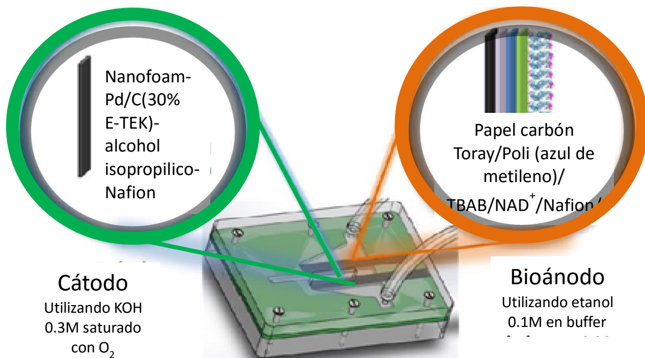
Figura 4.6.4.1. Diagrama de la celda híbrida Alcohol deshidrogenasa/Paladio
