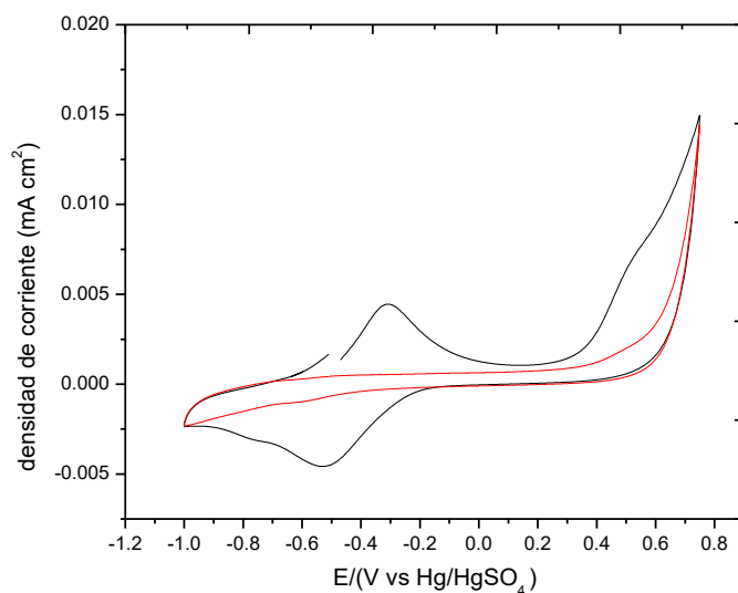
Figura 3.3.5.2. Voltamperometria cíclica de bioánodo desarrollado sin la capa de Nafion-agua.
