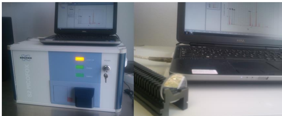
Figura 4.4.1 Equipo de Fluorescencia de Rayos X.
