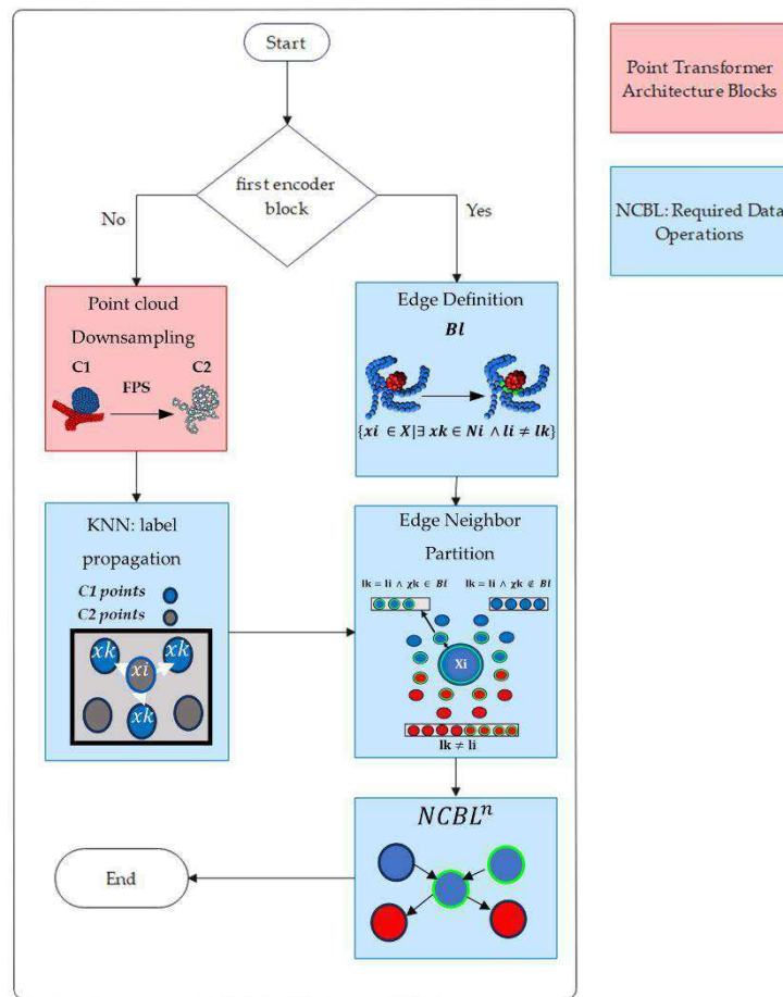
Figura 6.7. Nested Contrastive Boundary Learning Point Transformer (NCBL-PT): Diagrama de flujo que muestra lo que sucede en cada bloque para llegar a los cálculos del NCBL. Imagen propia.
